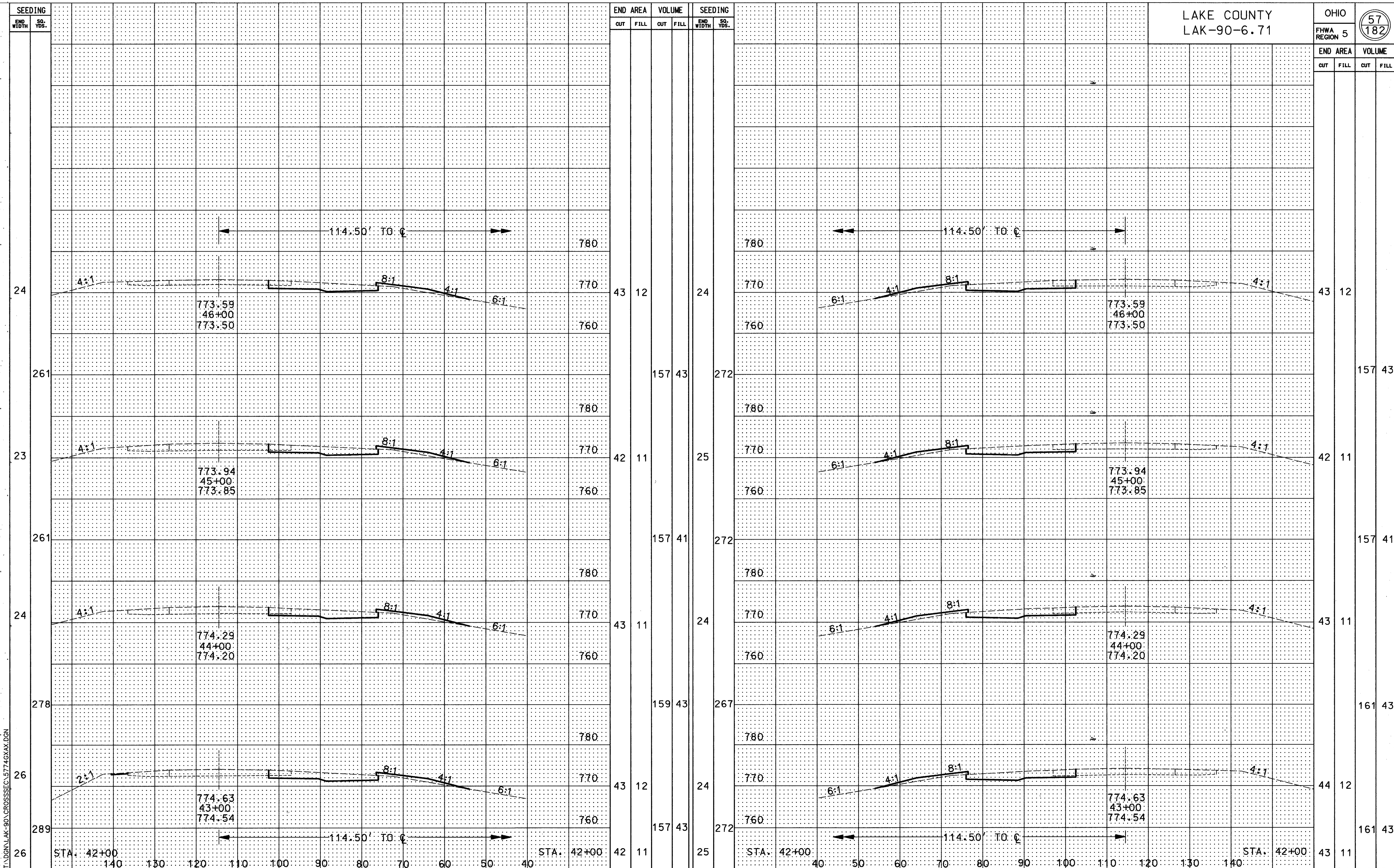
CROSS SECTIONS STA. 43+00 TO STA. 46+00 (WB) & STA. 43+00 TO STA. 46+00 (EB)
