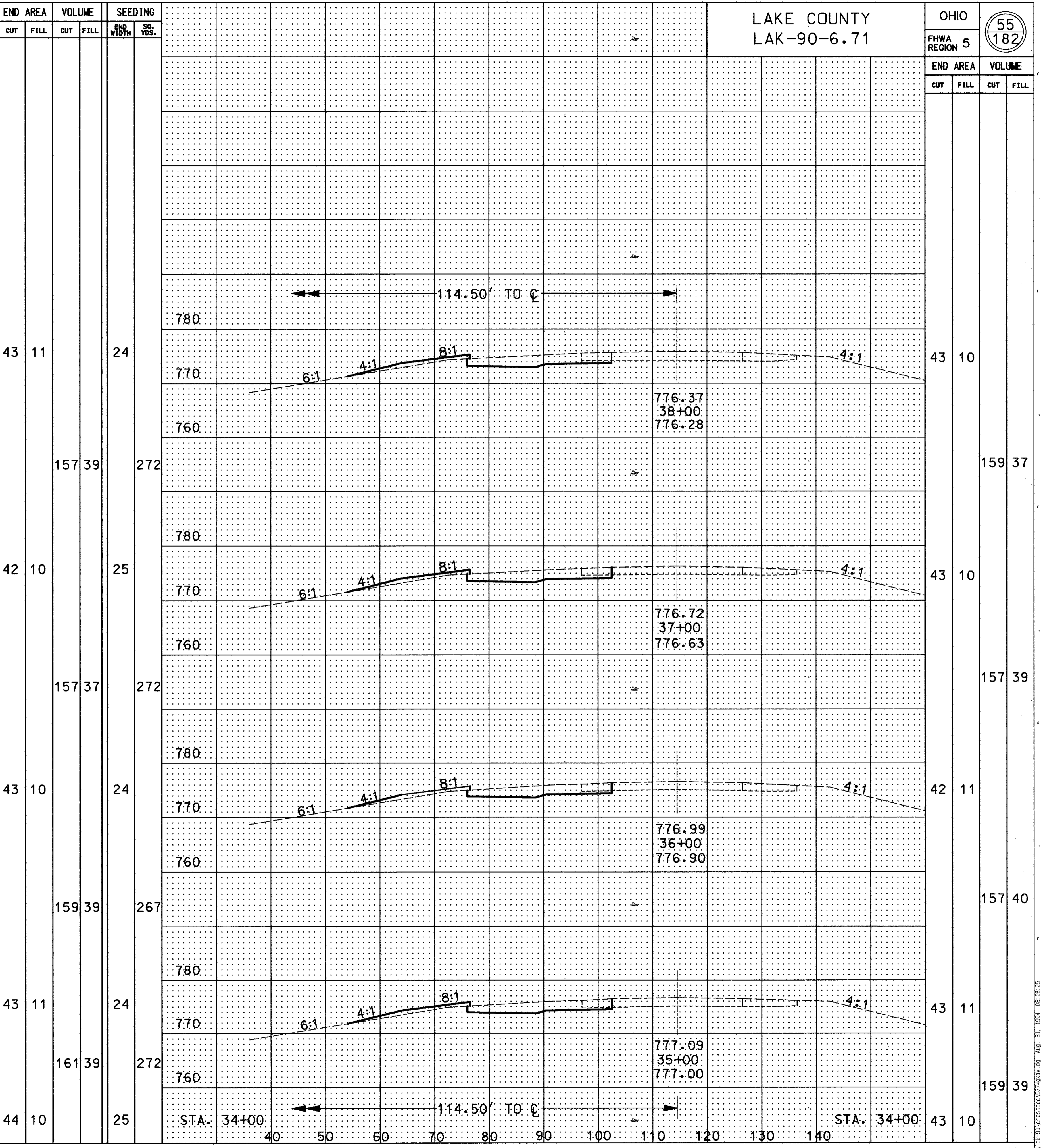
CROSS SECTIONS STA. 35+00 TO STA. 38+00 (WB) & STA. 35+00 TO STA. 38+00 (EB)
