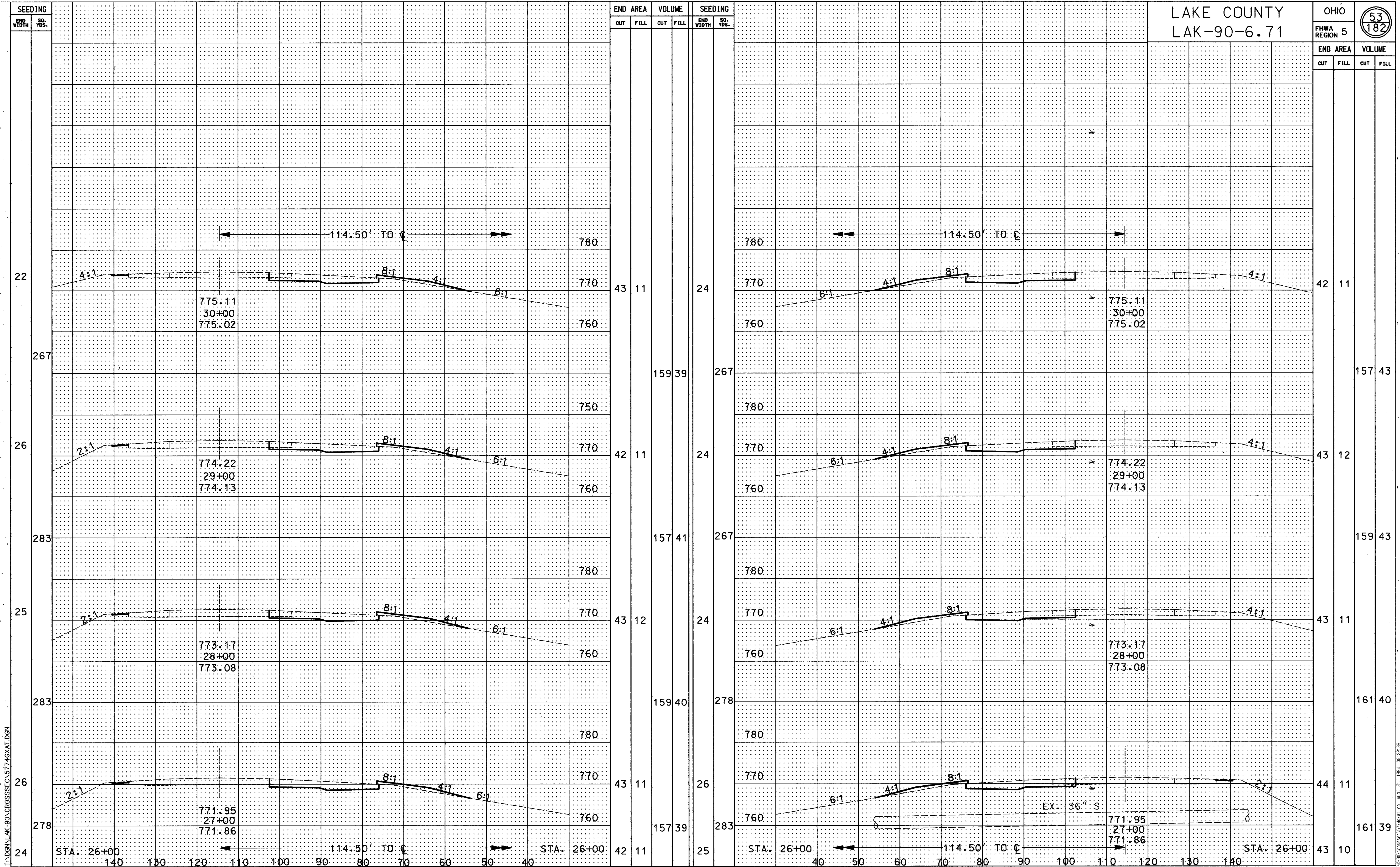
CROSS SECTIONS STA. 27+00 TO STA. 30+00 (WB) & STA. 27+00 TO STA. 30+00 (EB)
