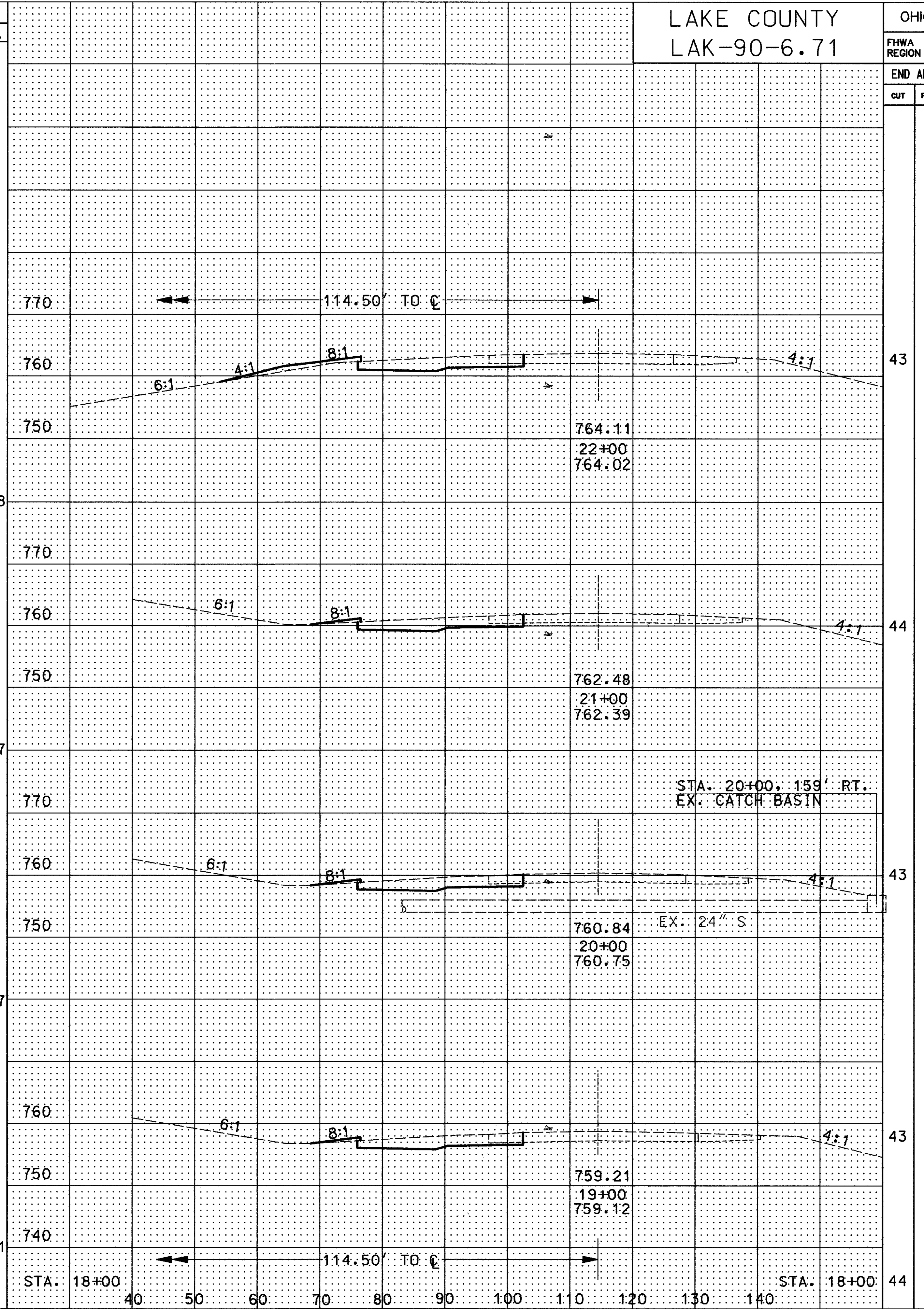
CROSS SECTIONS STA. 19+00 TO STA. 22+00 (WB) & STA. 19+00 TO STA. 22+00 (EB)
