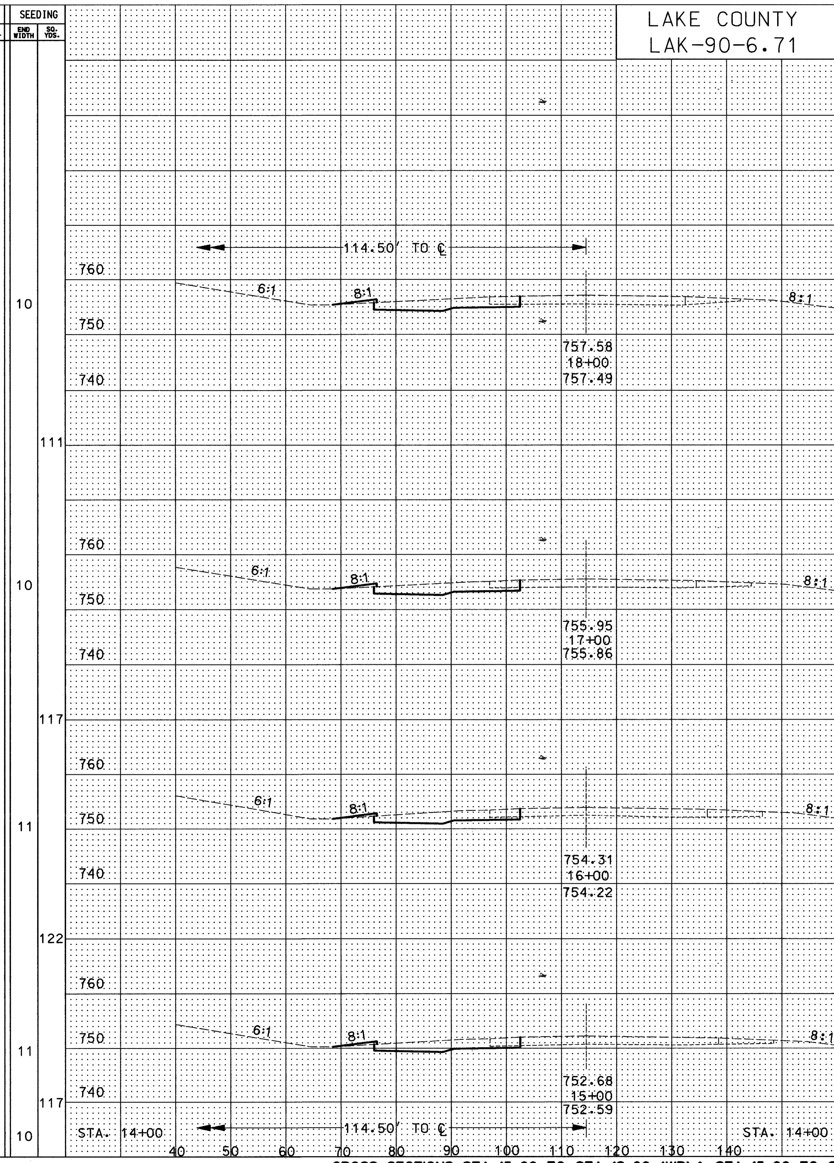
CROSS SECTIONS STA. 15+00 TO STA. 18+00 (WB) & STA. 15+00 TO STA. 18+00 (EB)
