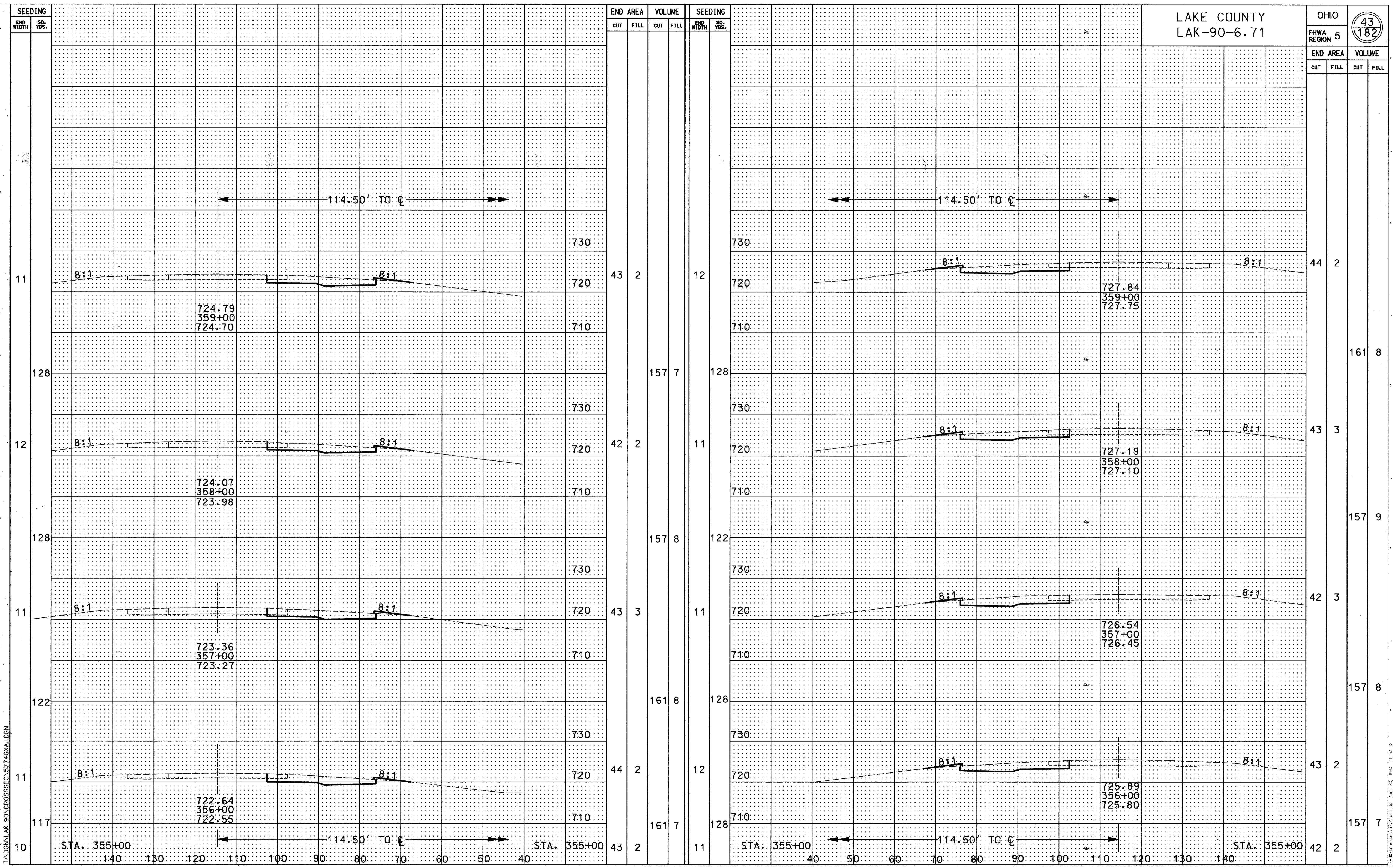
CROSS SECTIONS STA. 356+00 TO STA. 359+00 (WB) & STA. 356+00 TO STA. 359+00 (EB)
