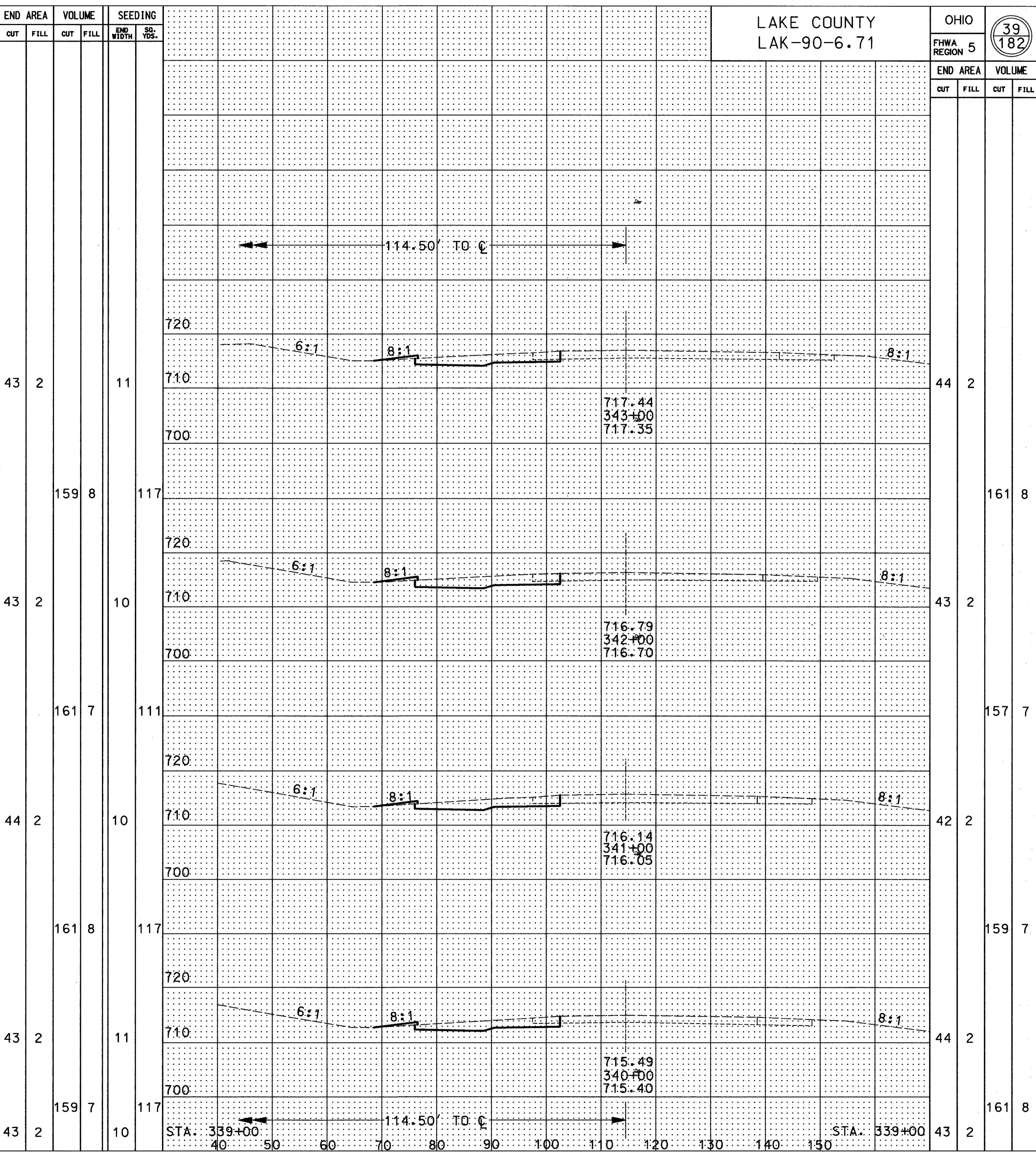
CROSS SECTIONS STA. 340+00 TO STA. 343+00 (WB) & STA. 340+00 TO STA. 343+00 (EB)
