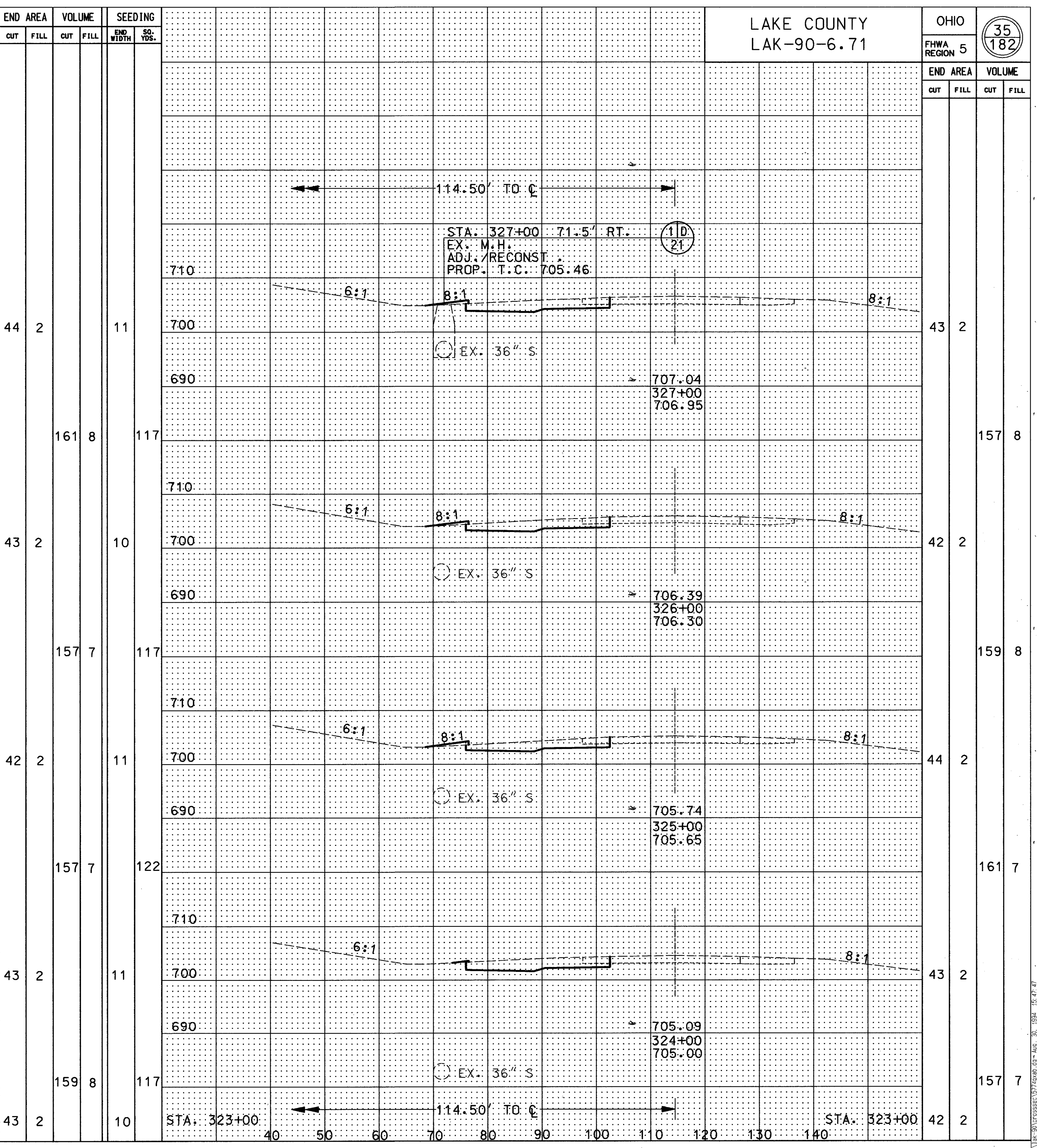
CROSS SECTIONS STA. 324+00 TO STA. 327+00 (WB) STA. 324+00 TO STA. 327+00 (EB)
