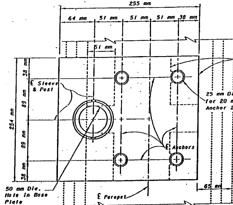
PLAN BP-2
