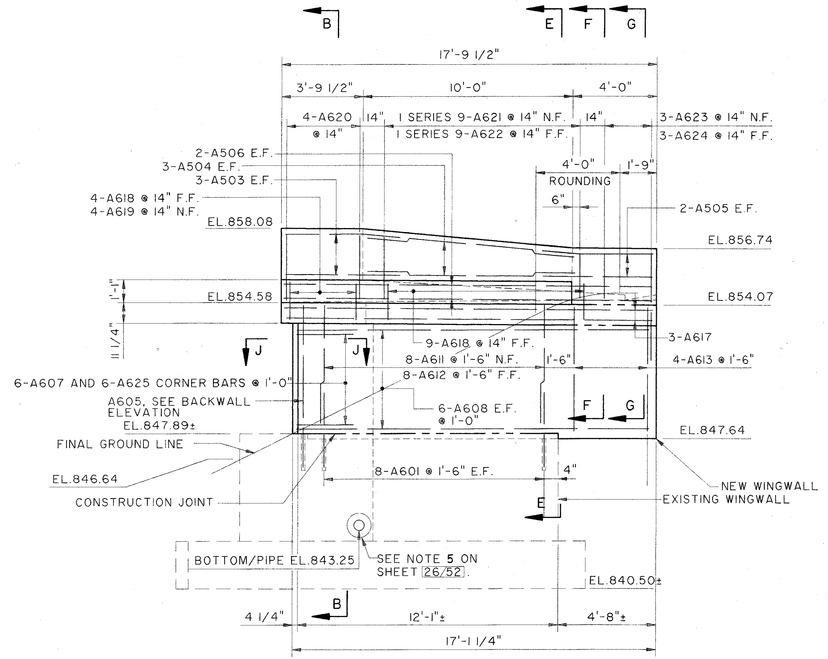
ELEVATION D-D
