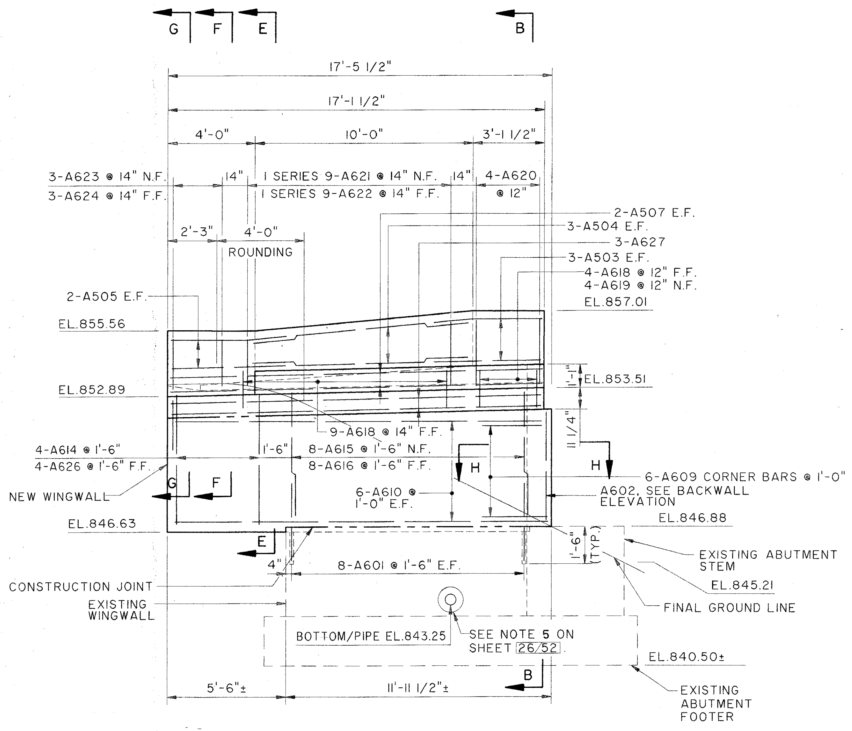
ELEVATION C-C
