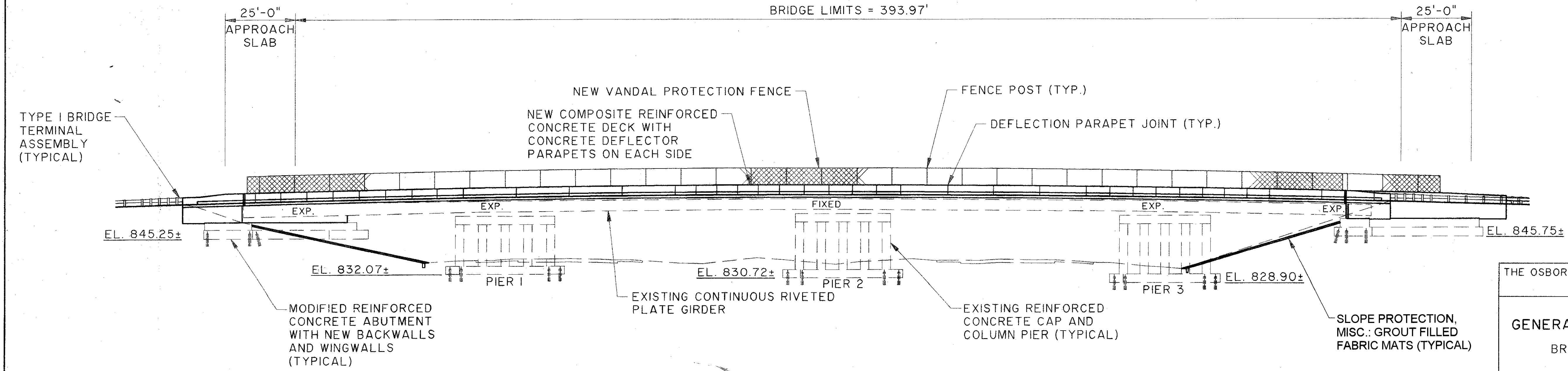
ELEVATION
