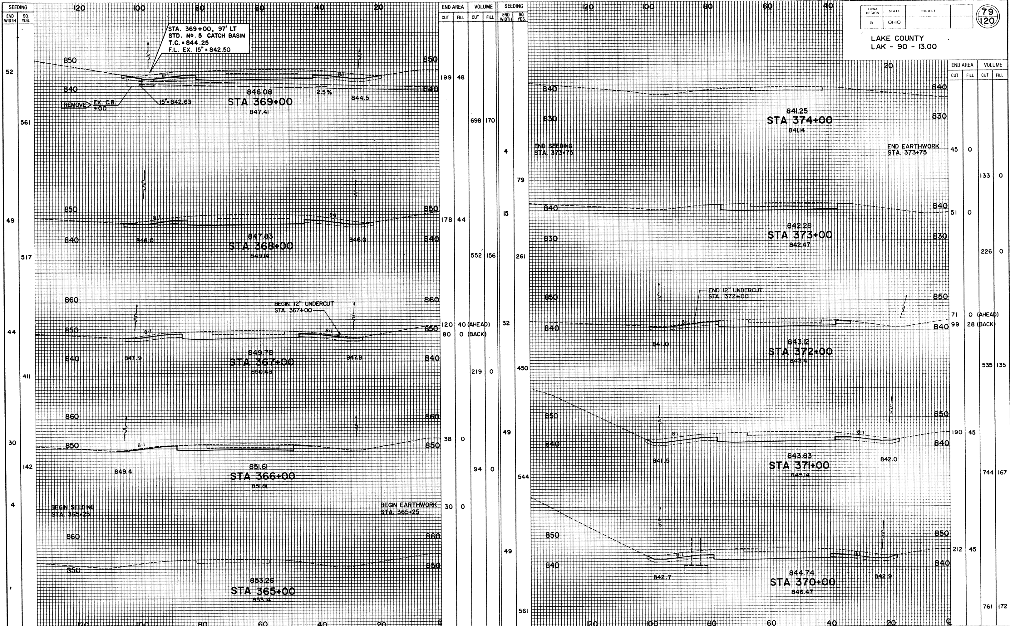
I-90 WESTBOUND - STA 365+00 TO STA 374+00
