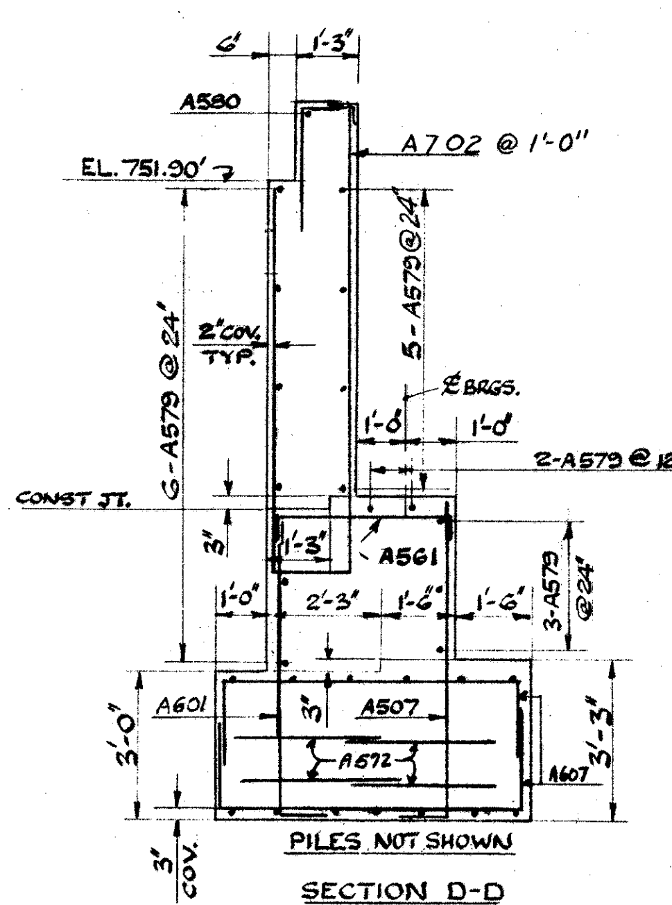
SECTION D-D
