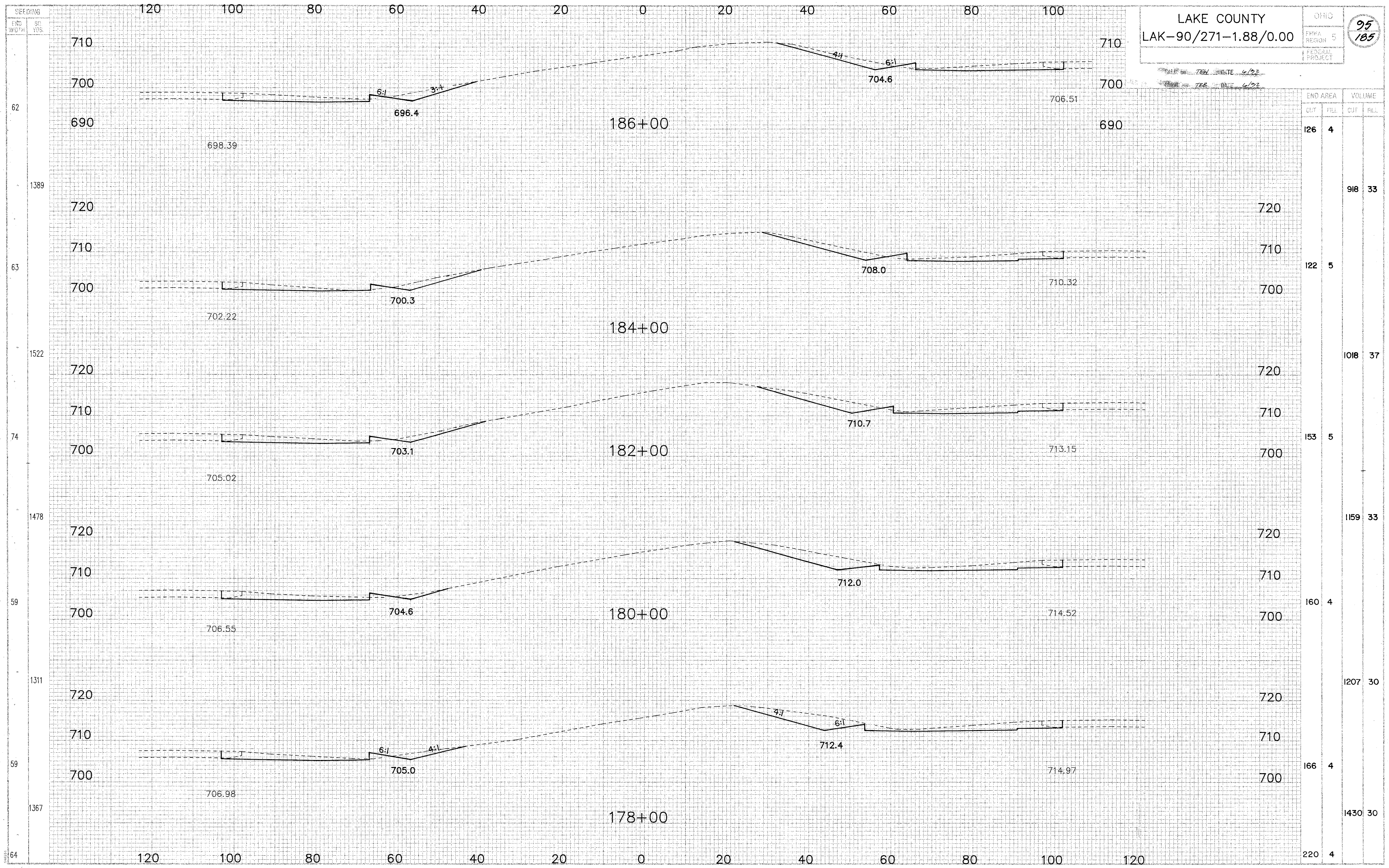
CROSS SECTIONS STA. 178+00 TO STA. 186+00
