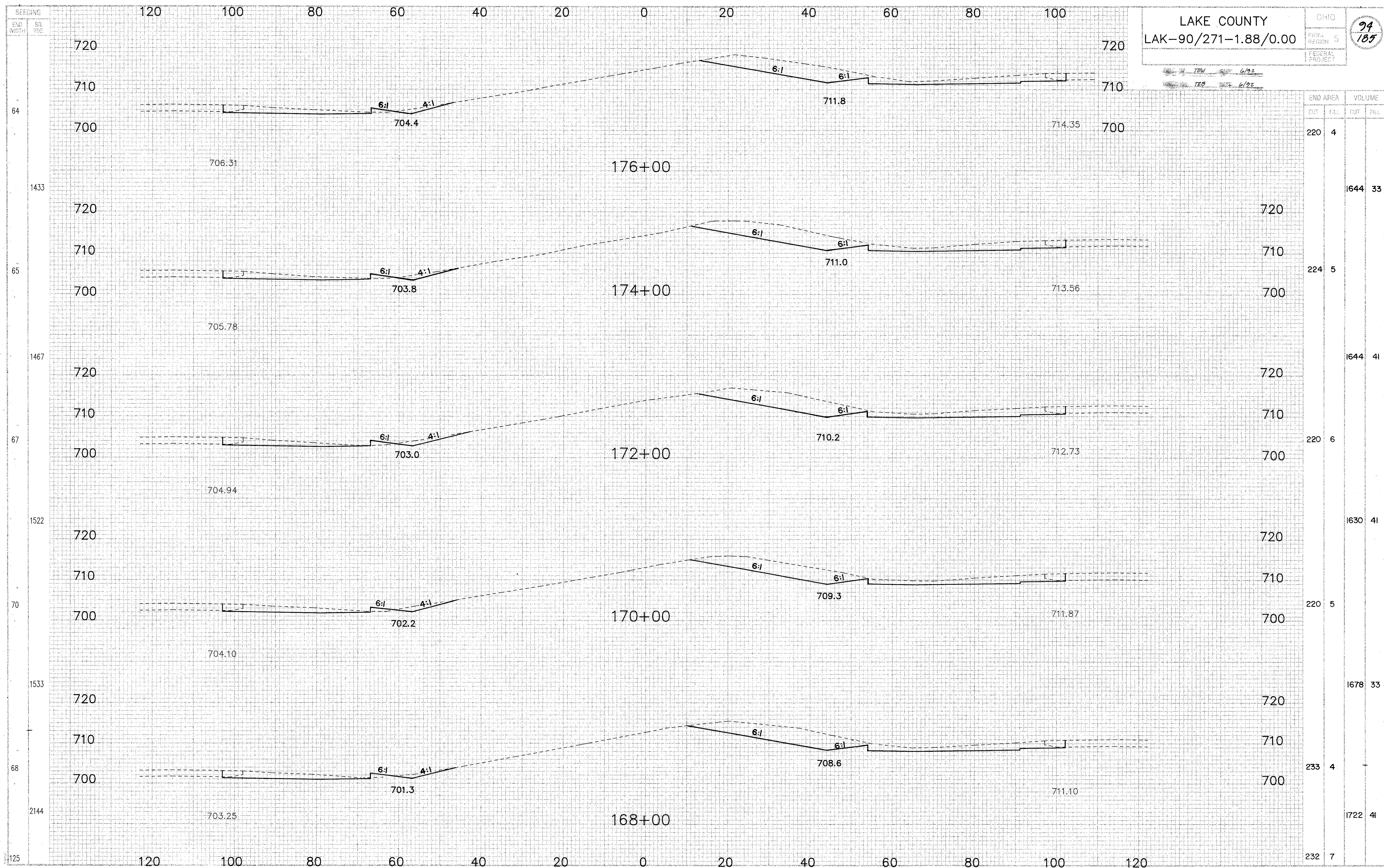
CROSS SECTIONS STA. 168+00 TO STA. 176+00
