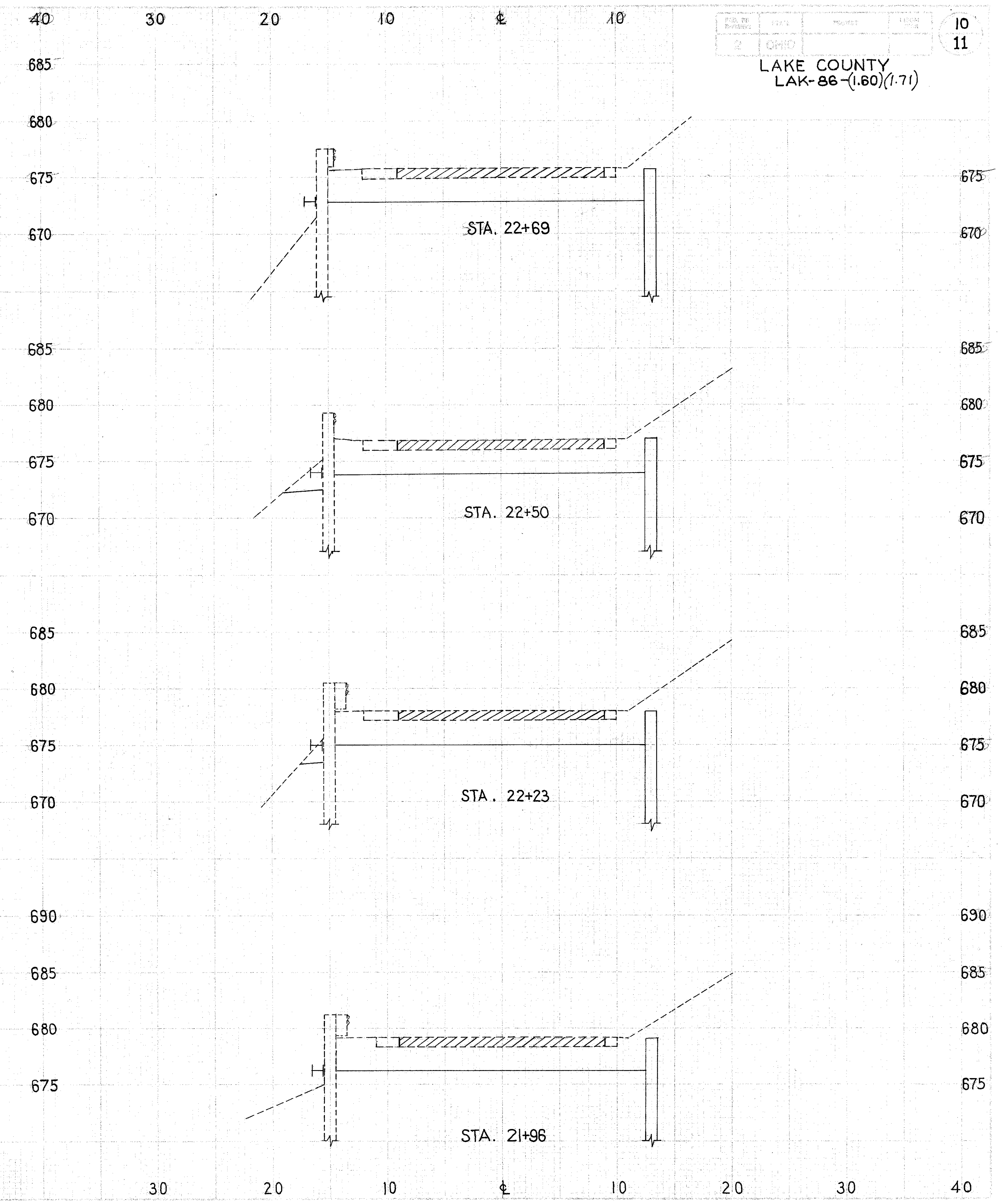
CROSS SECTIONS S.R. 86 STA. 21+05 TO STA. 22+69
