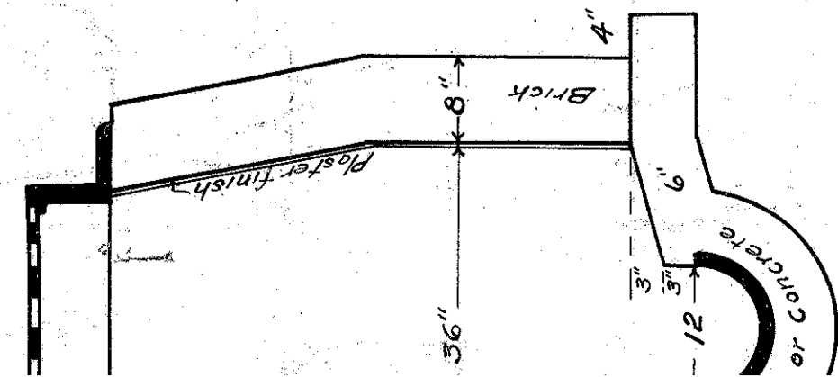
SECTION MANHOLE.
