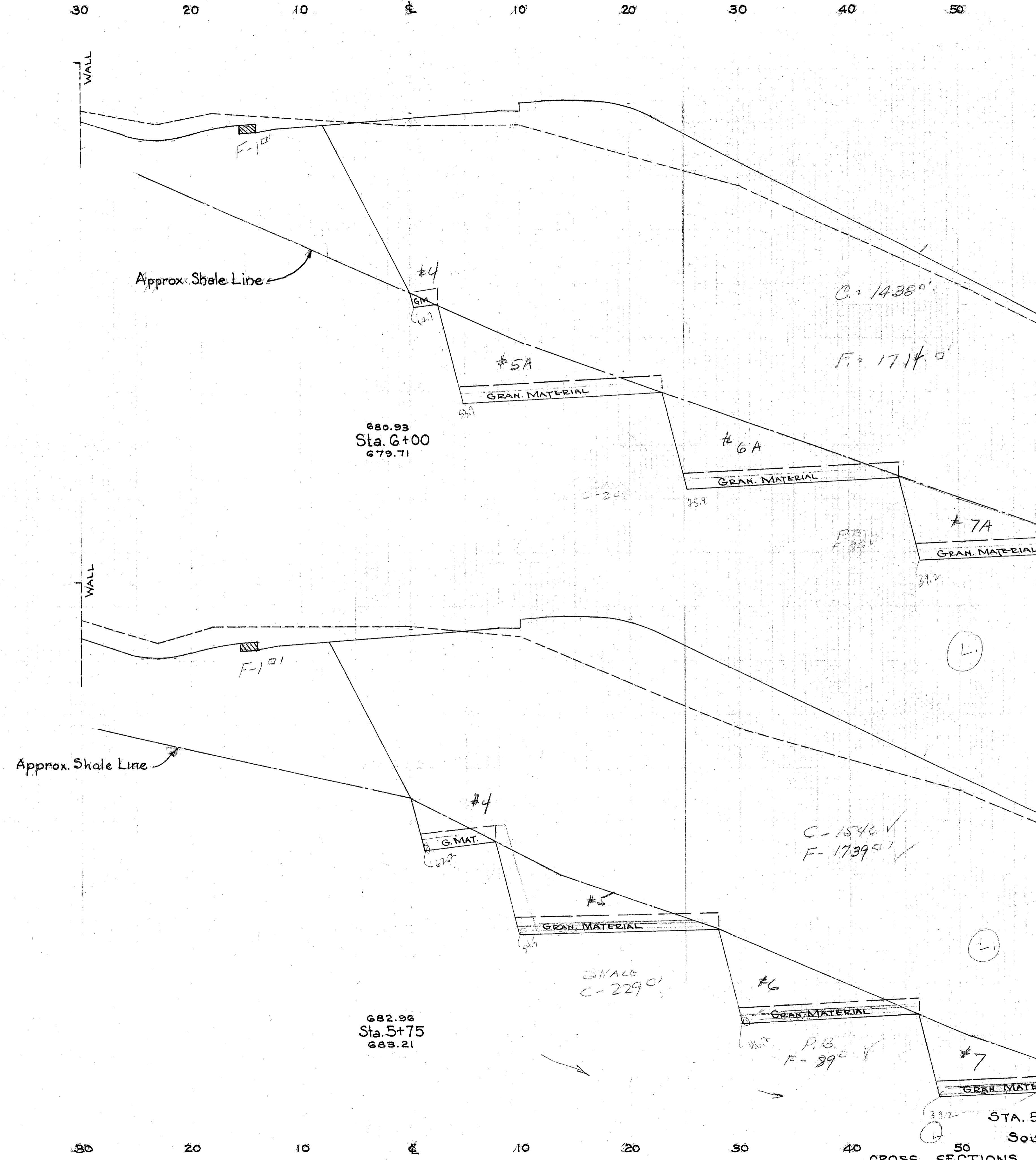
CROSS SECTIONS STA. 5+75 TO STA. G+00
