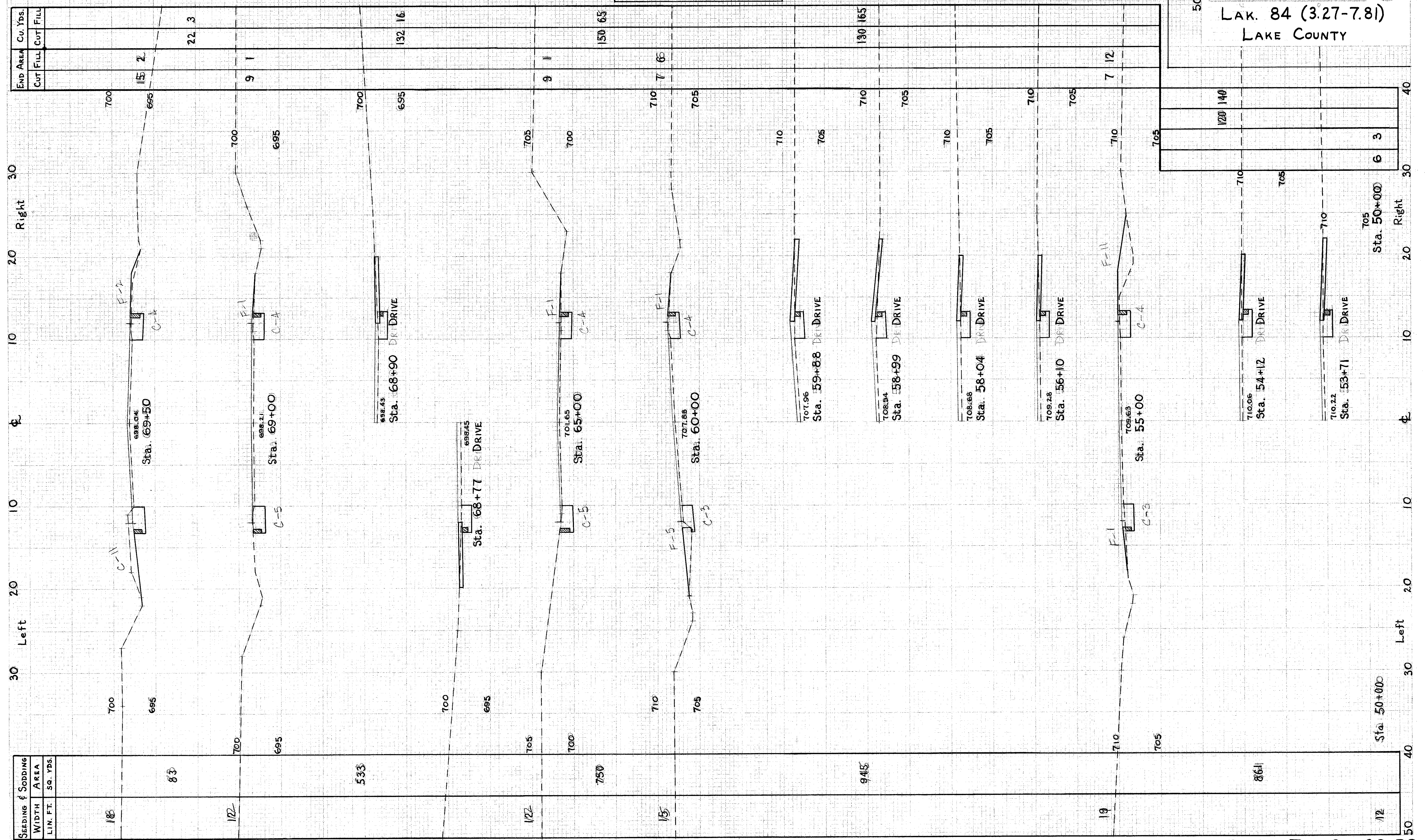
X SECTIONS STA. 53+71 To STA. 69+50
