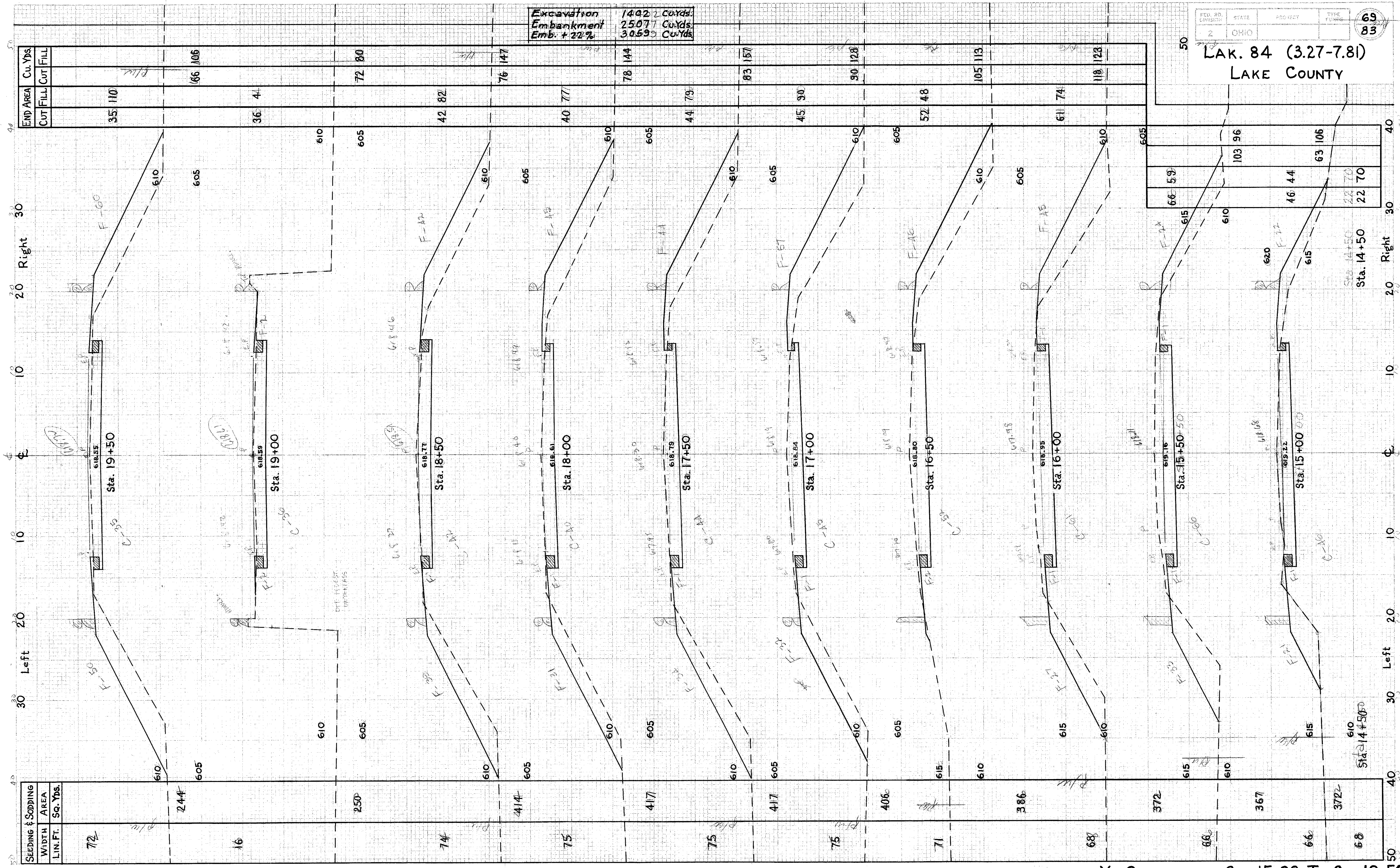
X SECTIONS STA. 15+00 TO STA. 19+50
