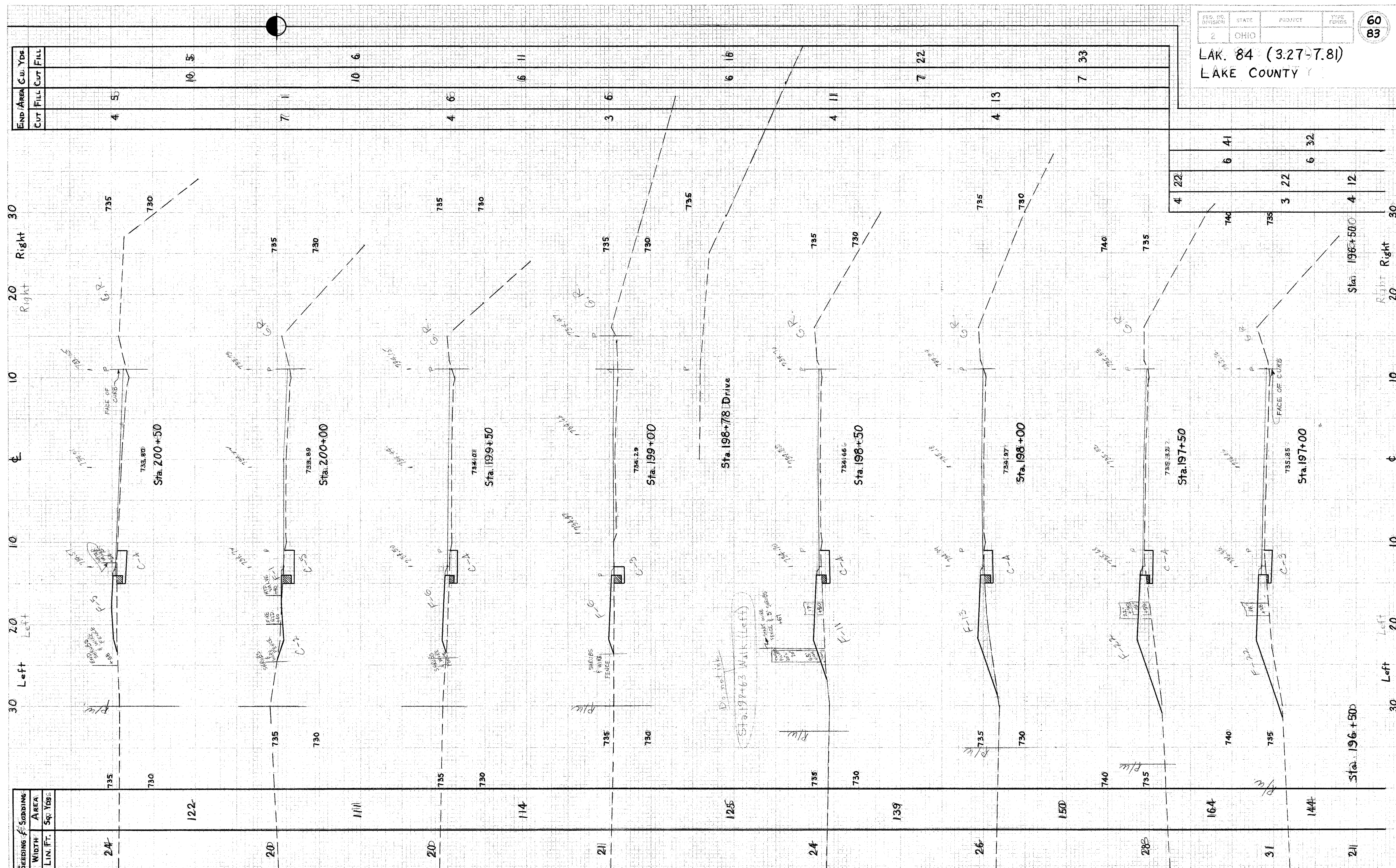
X SECTIONS STA. 197+00 To STA. 200+50
