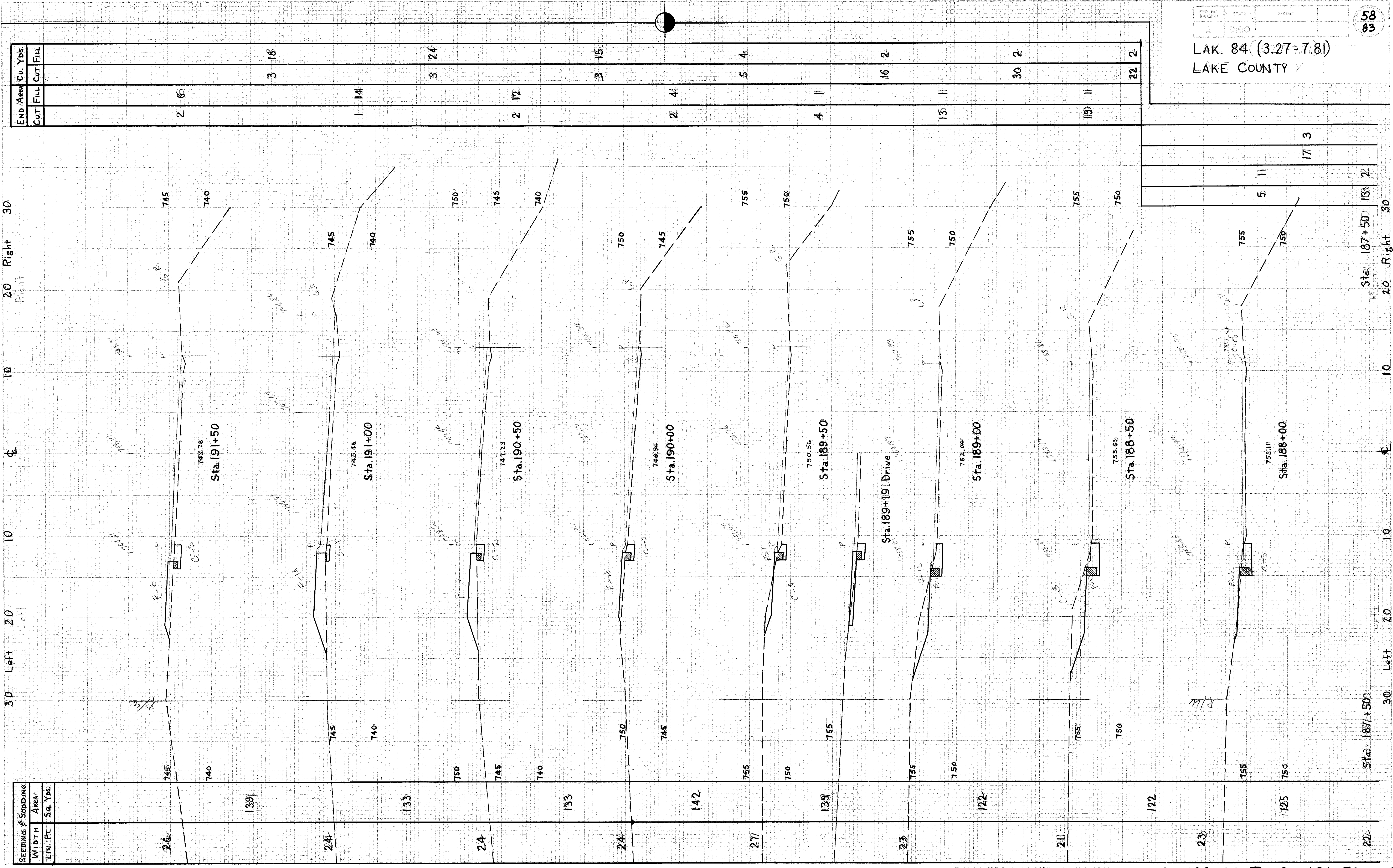
X SECTIONS STA. 188+00 To STA. 191+50
