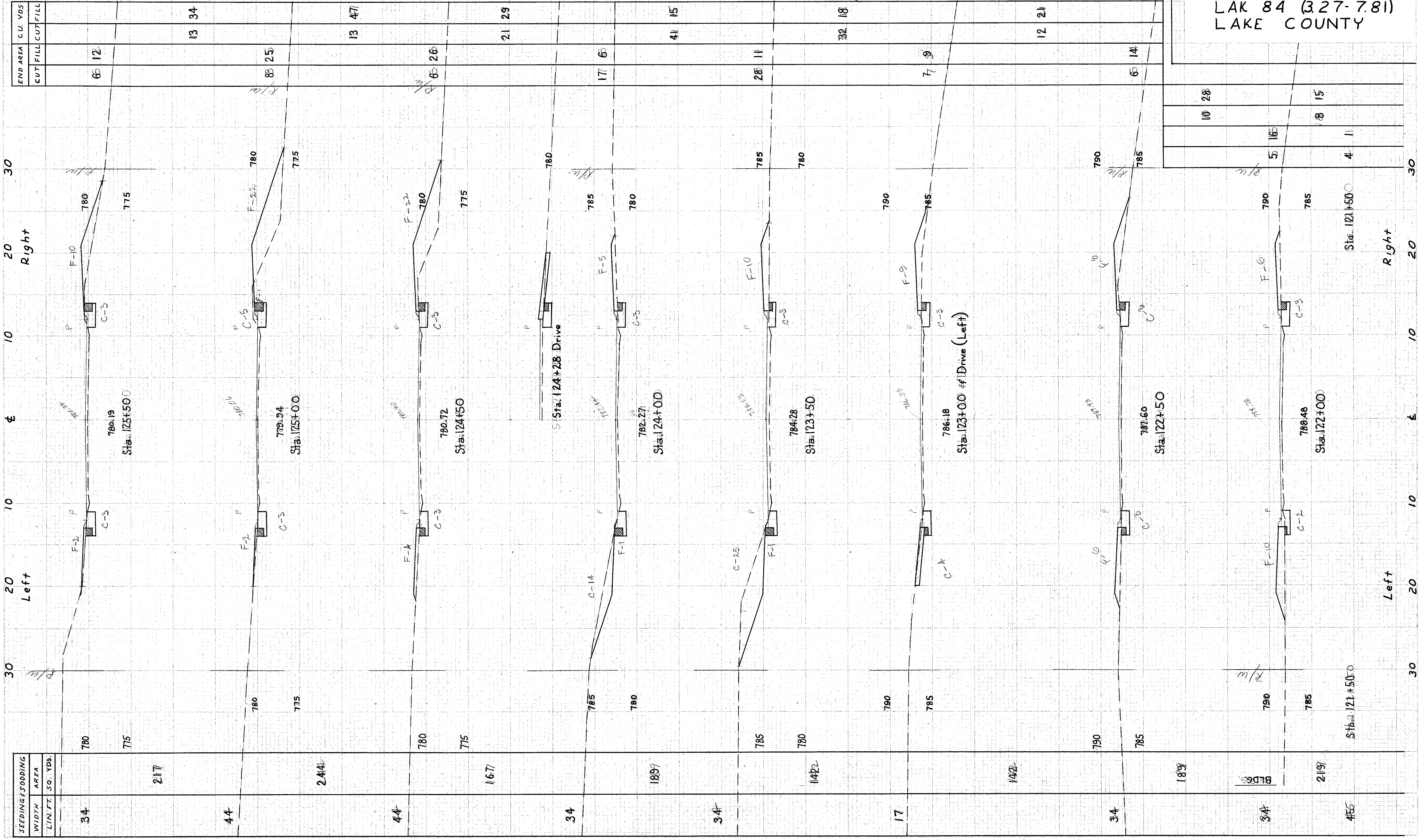
X SECTIONS STA. 122+00 To STA. 125+50
