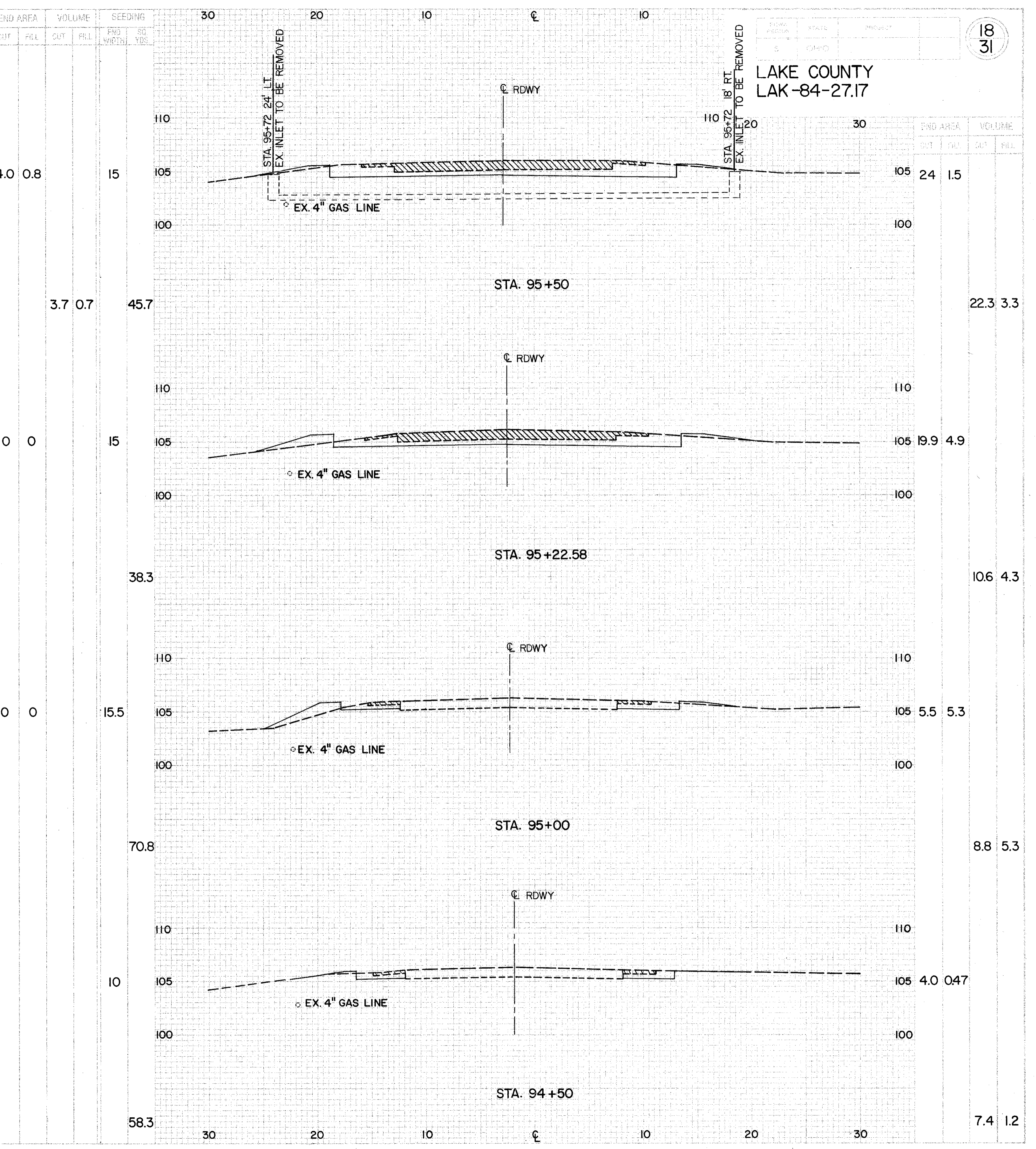
S.R. 84 X-SECTIONS STA. 93+00 TO STA. 95+50
