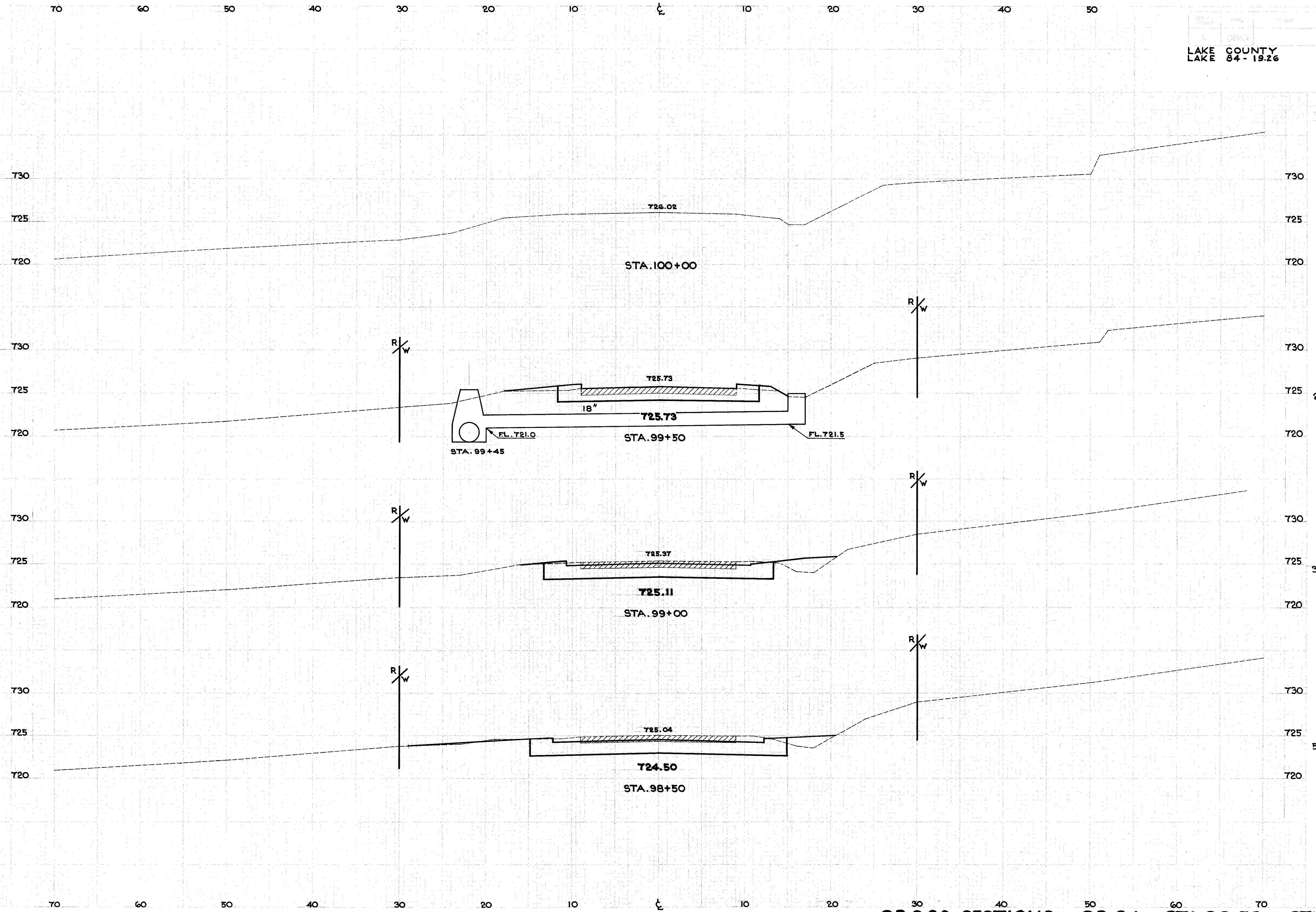
CROSS SECTIONS... S.R. 84... STA. 98+50 to STA. 100+00
