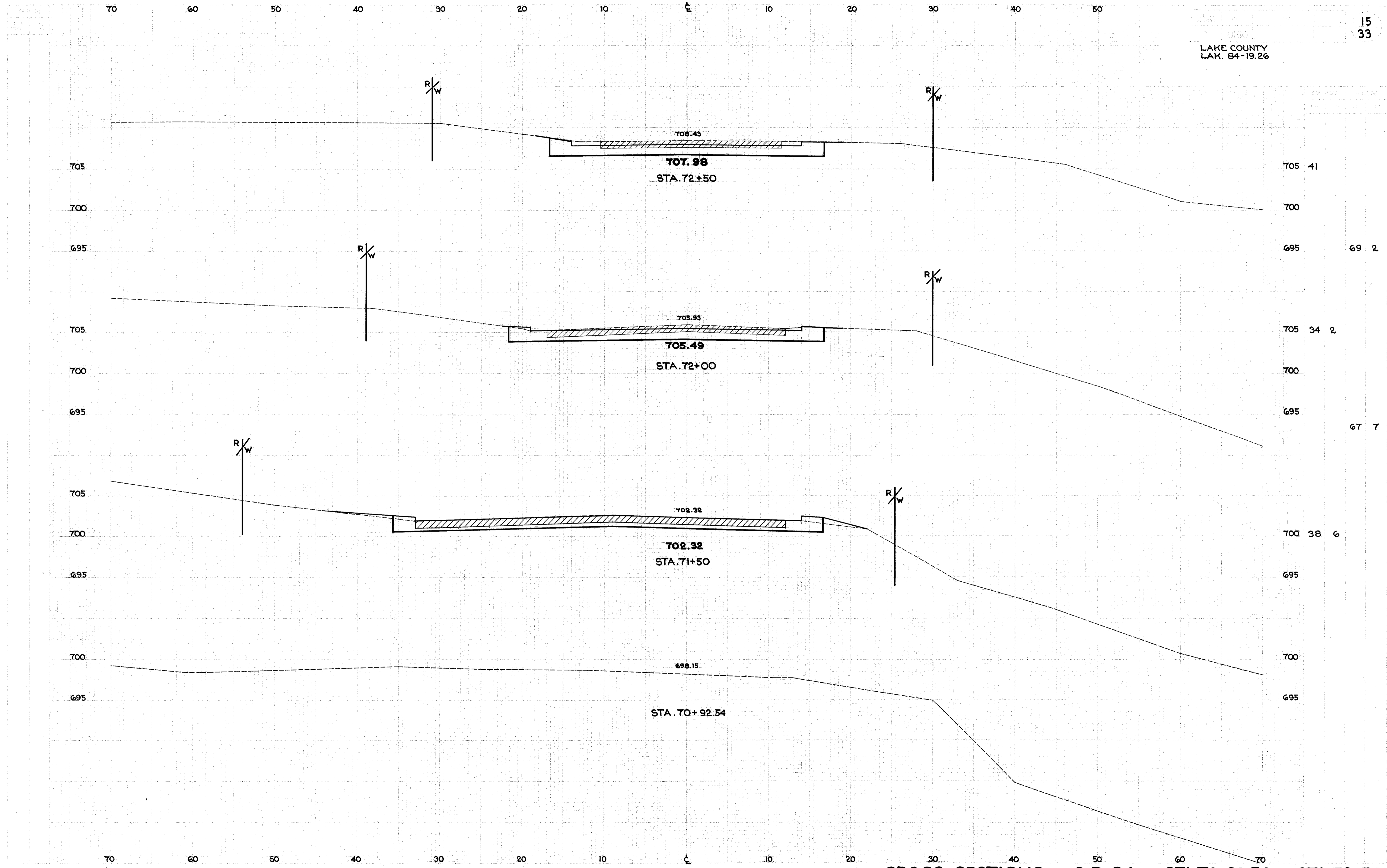
CROSS SECTIONS... S.R. 84... STA. 70+92.54 to STA. 72+50
