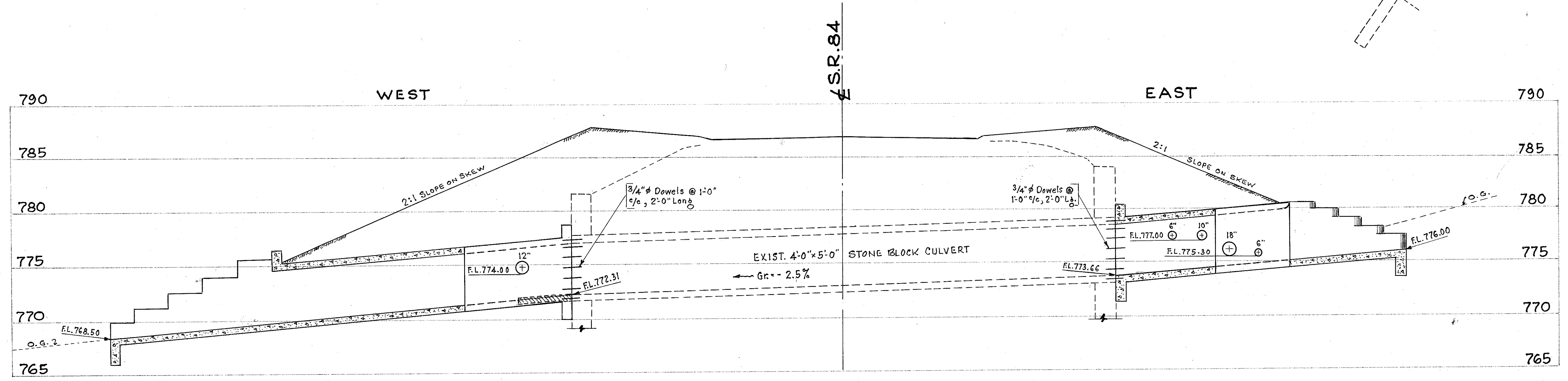
SECTION A-A
