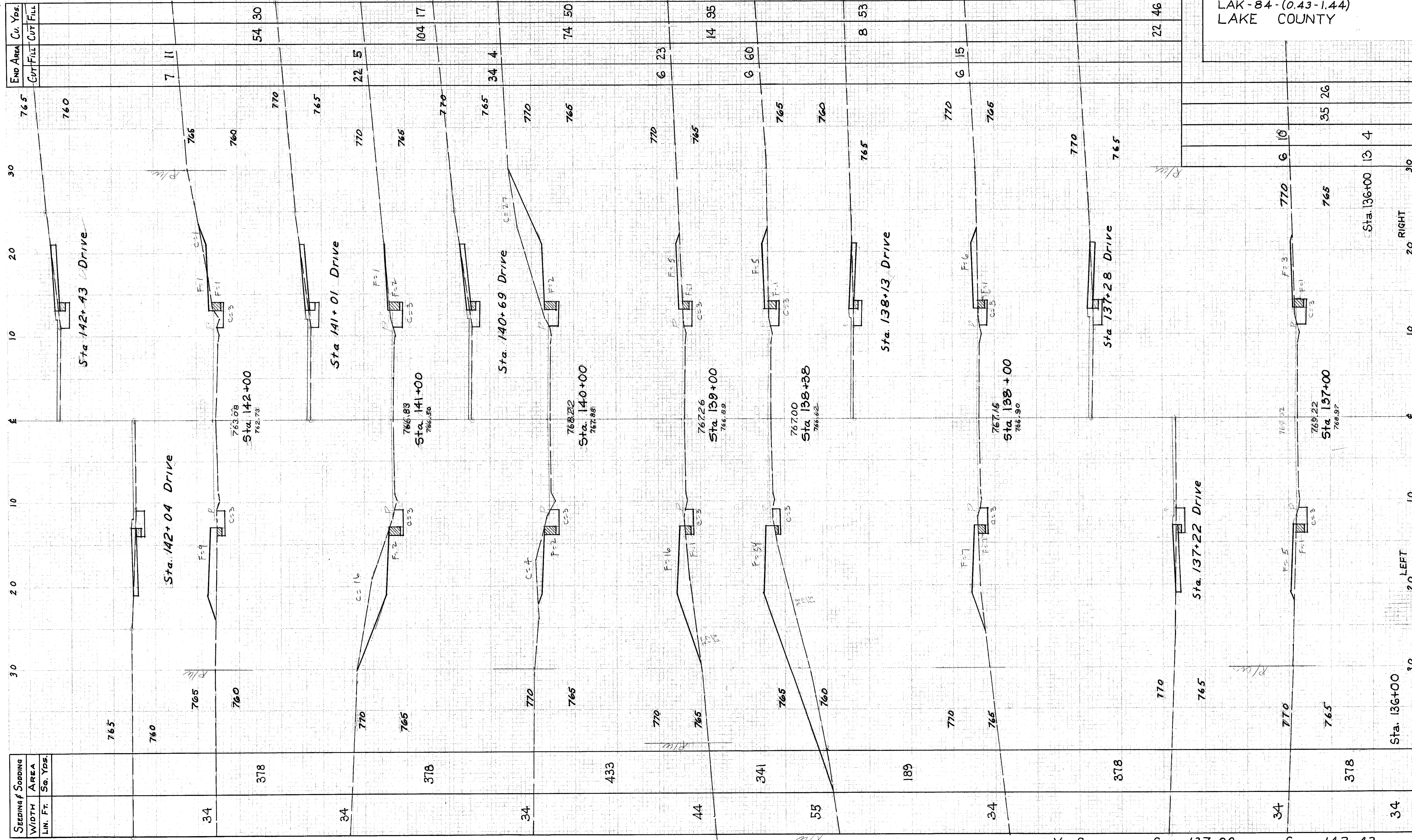
X-SECTIONS STA. 137+00 TO STA 142+43
