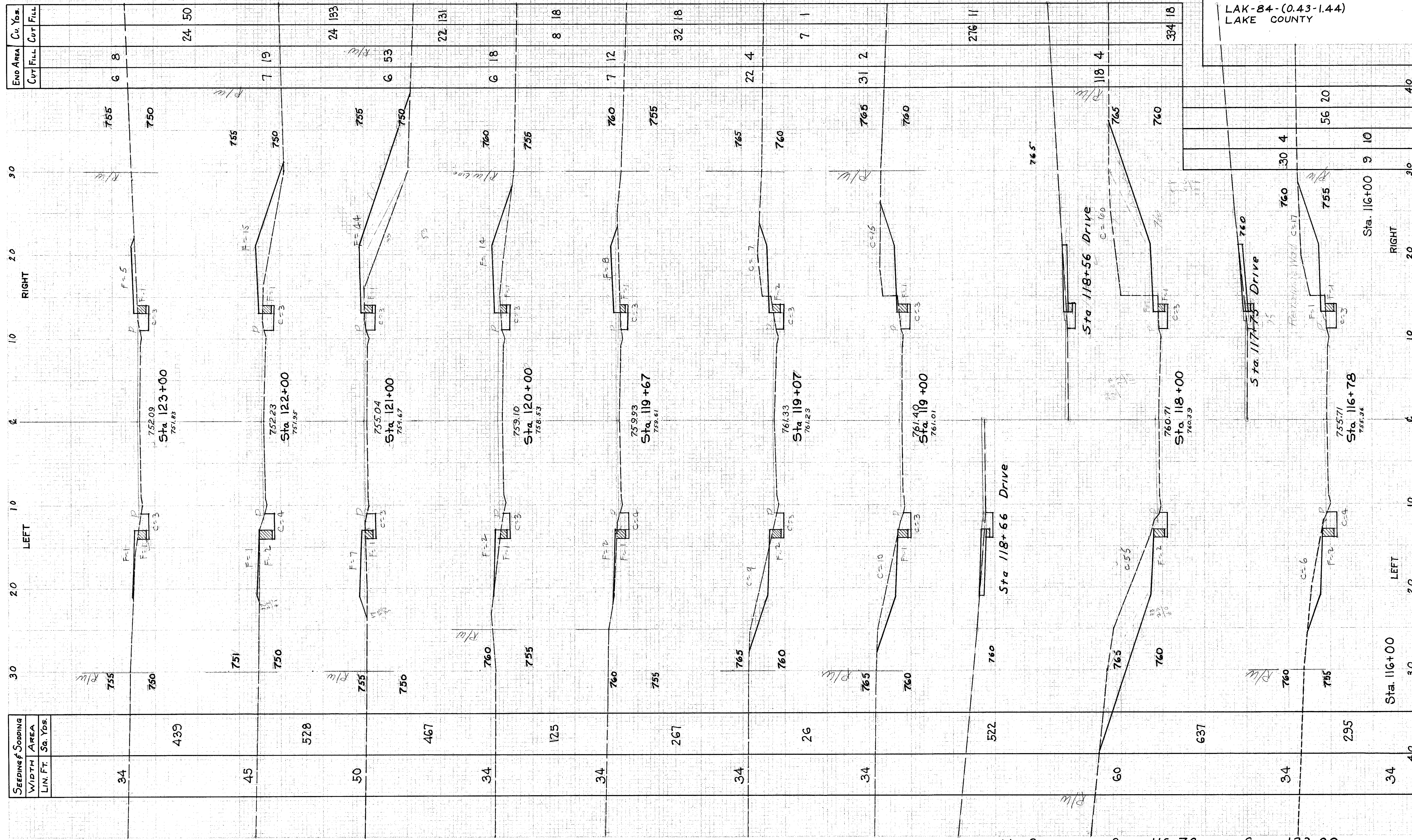
X- SECTIONS STA. 116+78 TO STA. 123+00
