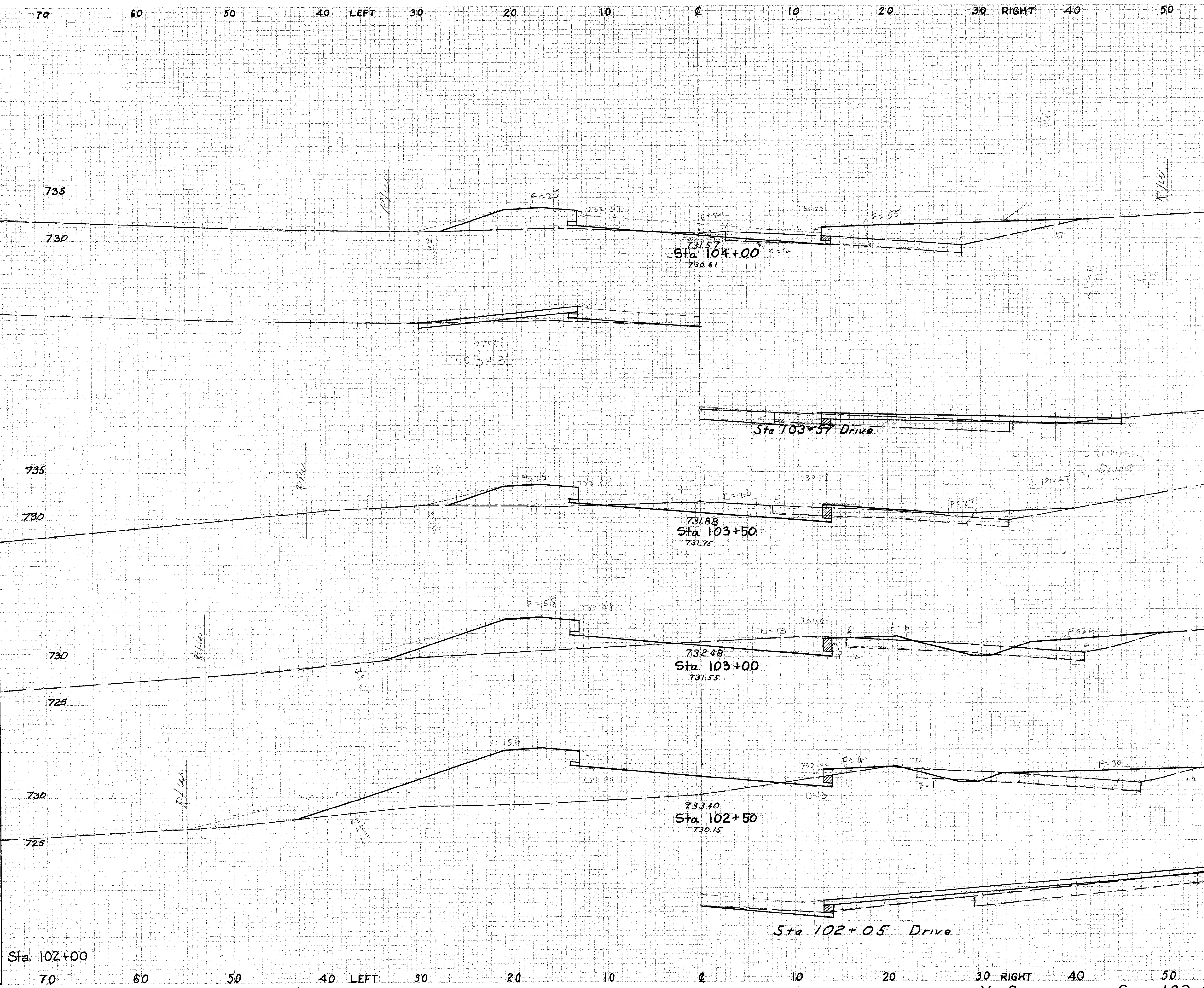
X-SECTIONS STA. 102+05 TO STA. 104+00
