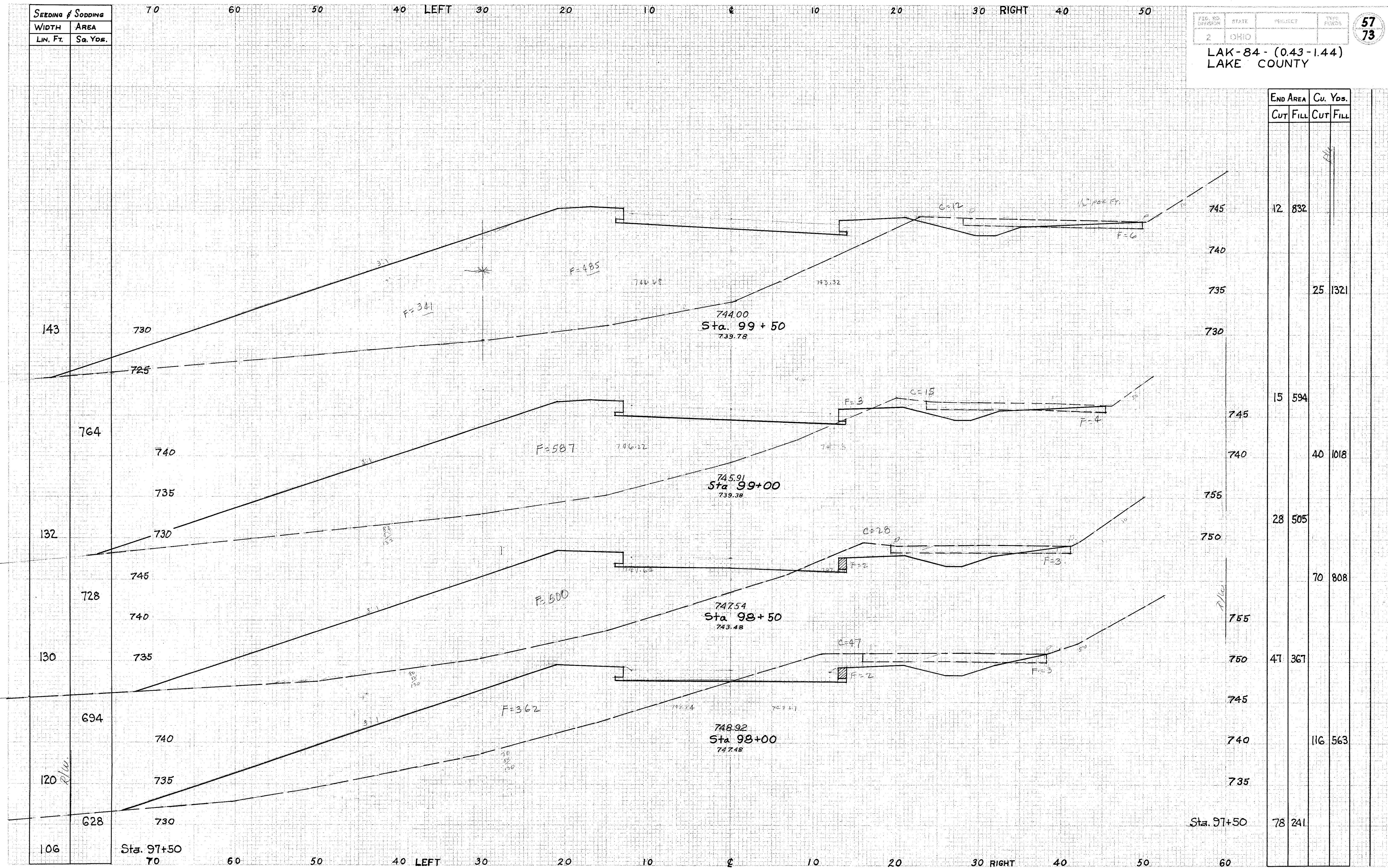
X-SECTIONS STA. 98+00 TO STA. 99+50
