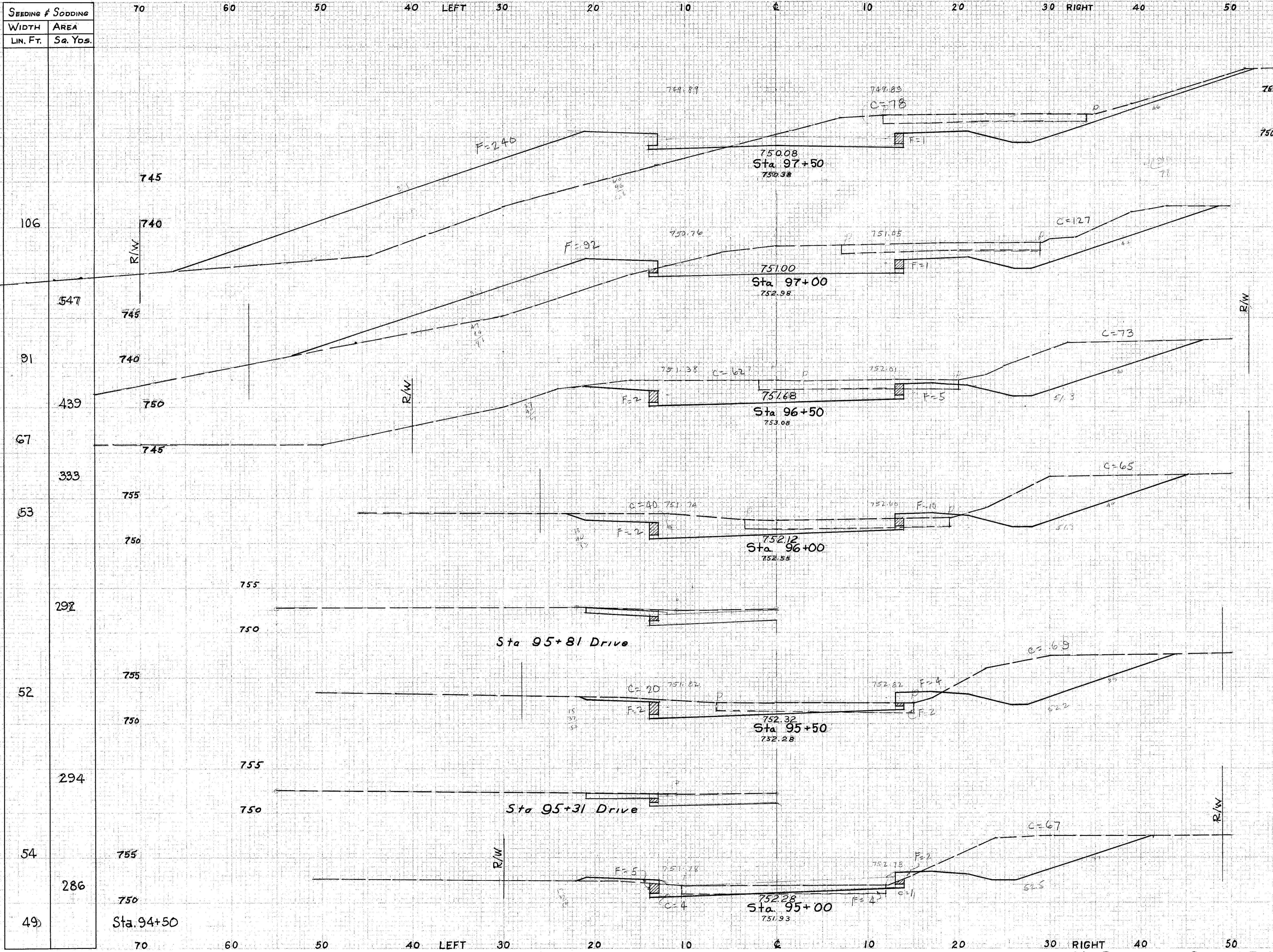
X-SECTIONS STA. 95+00 TO STA. 97+50
