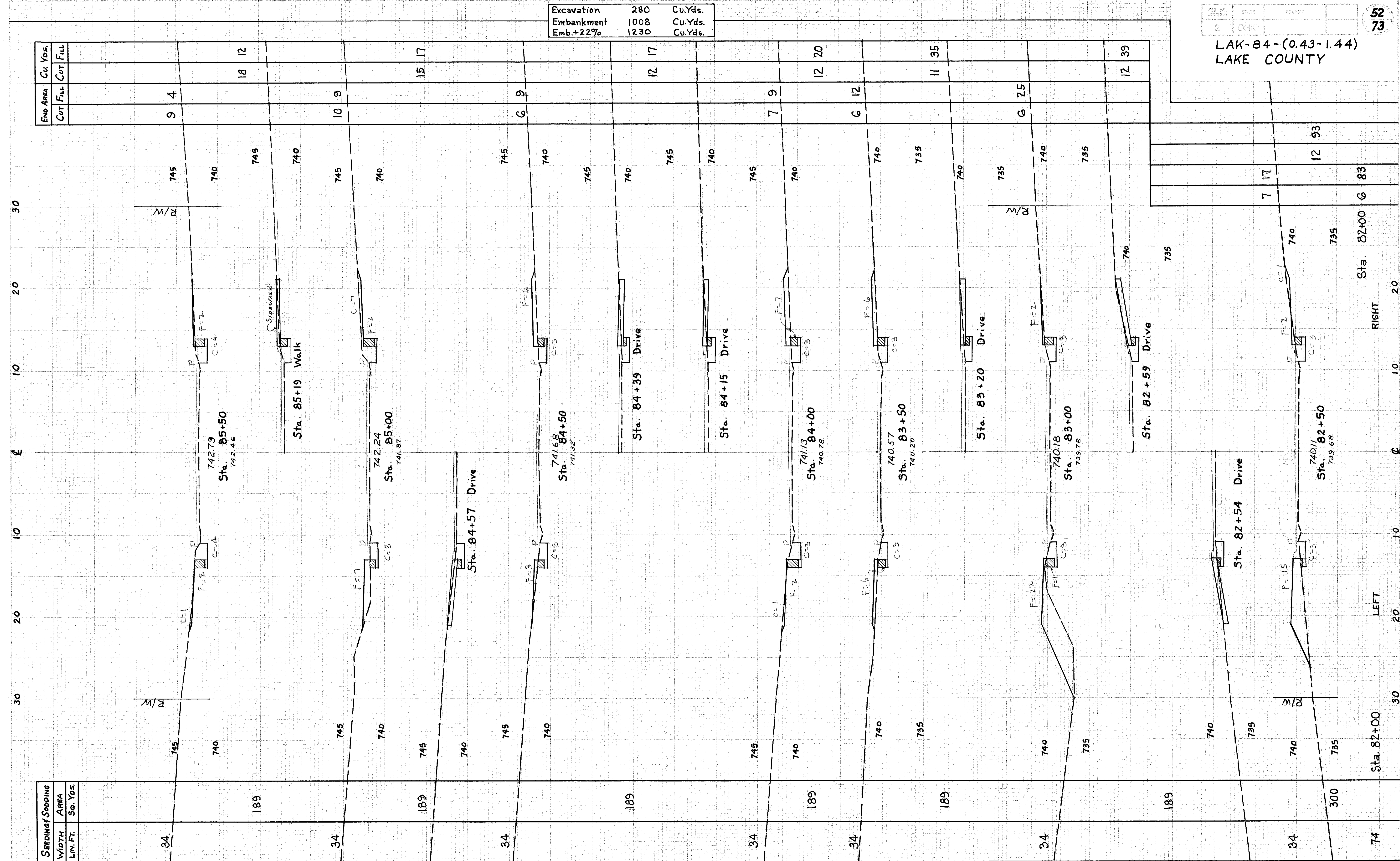
X-SECTIONS STA. 82+50 TO STA 85+50
