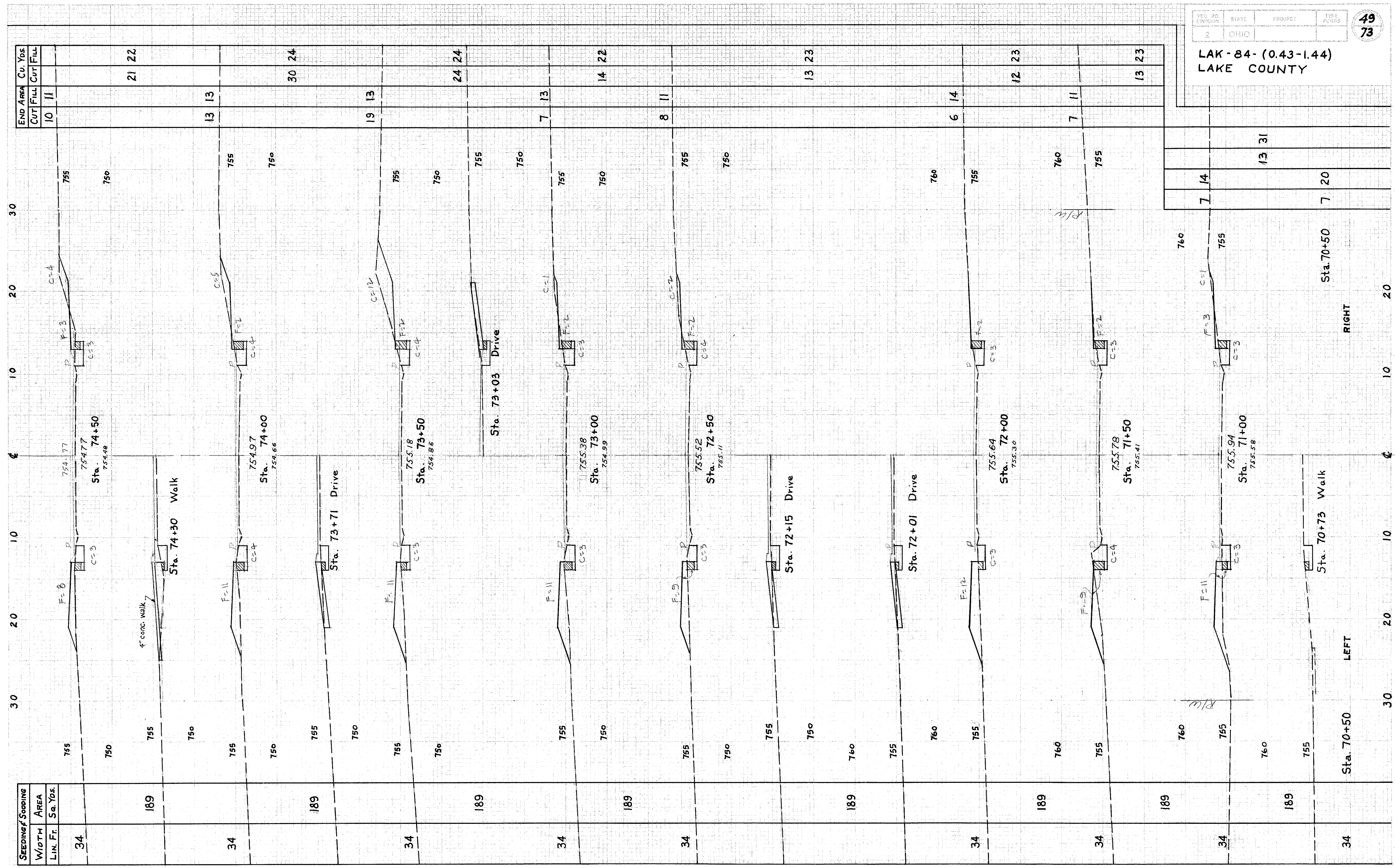
X-SECTIONS STA. 70+73 TO STA. 74+50
