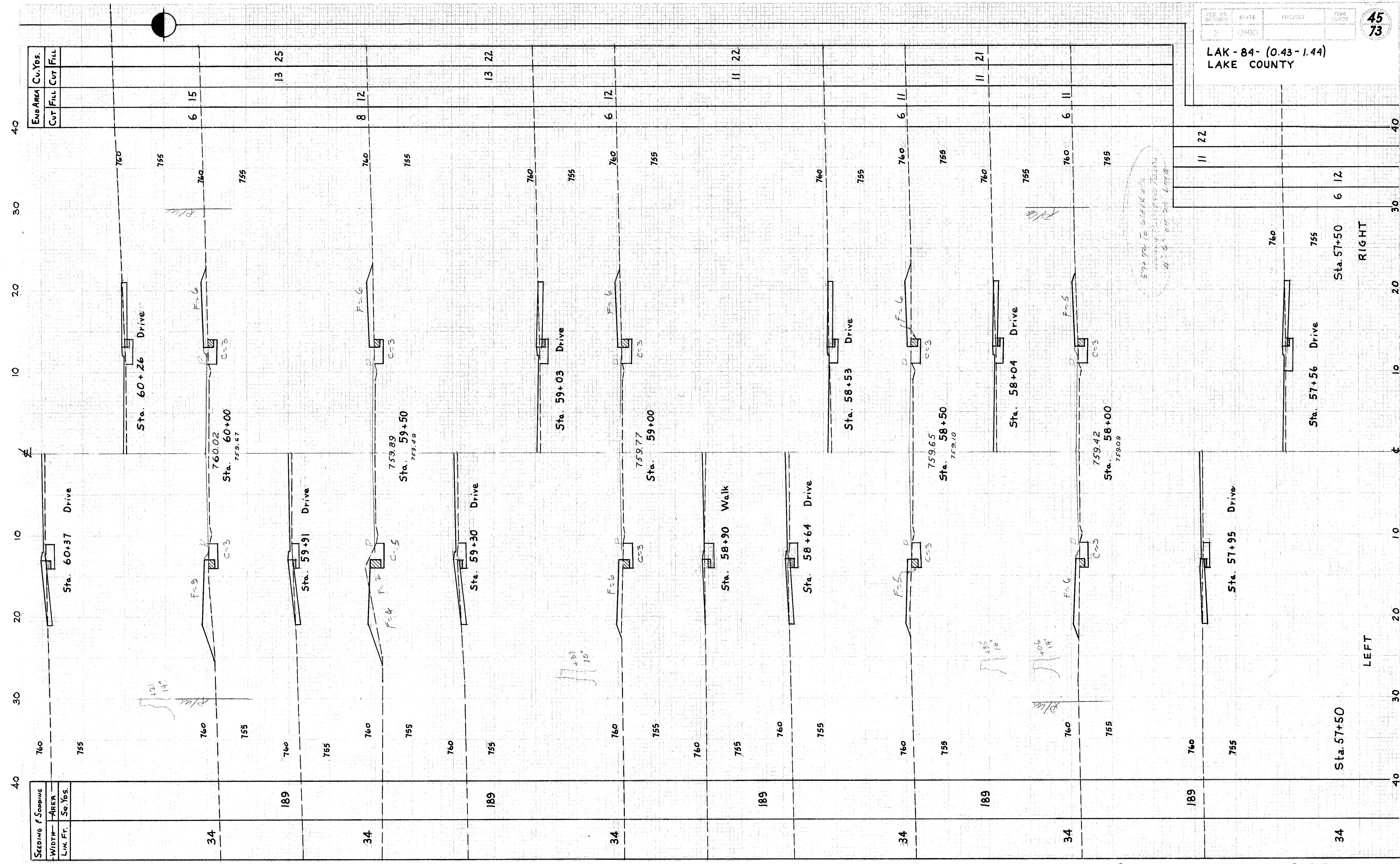
X-SECTIONS STA. 57+56 TO STA. 60+37
