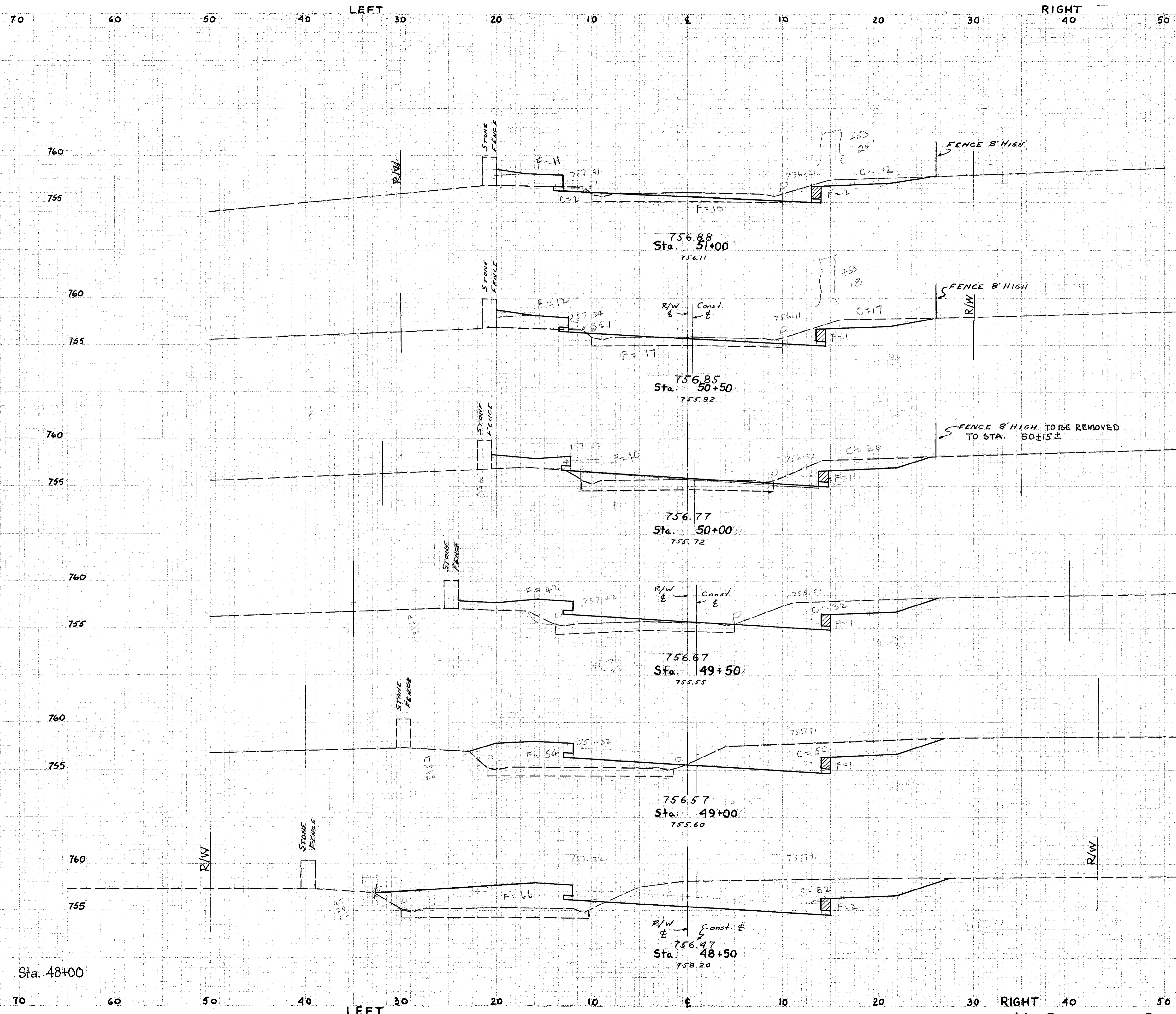
X-SECTIONS STA. 48+50 TO STA. 51+00
