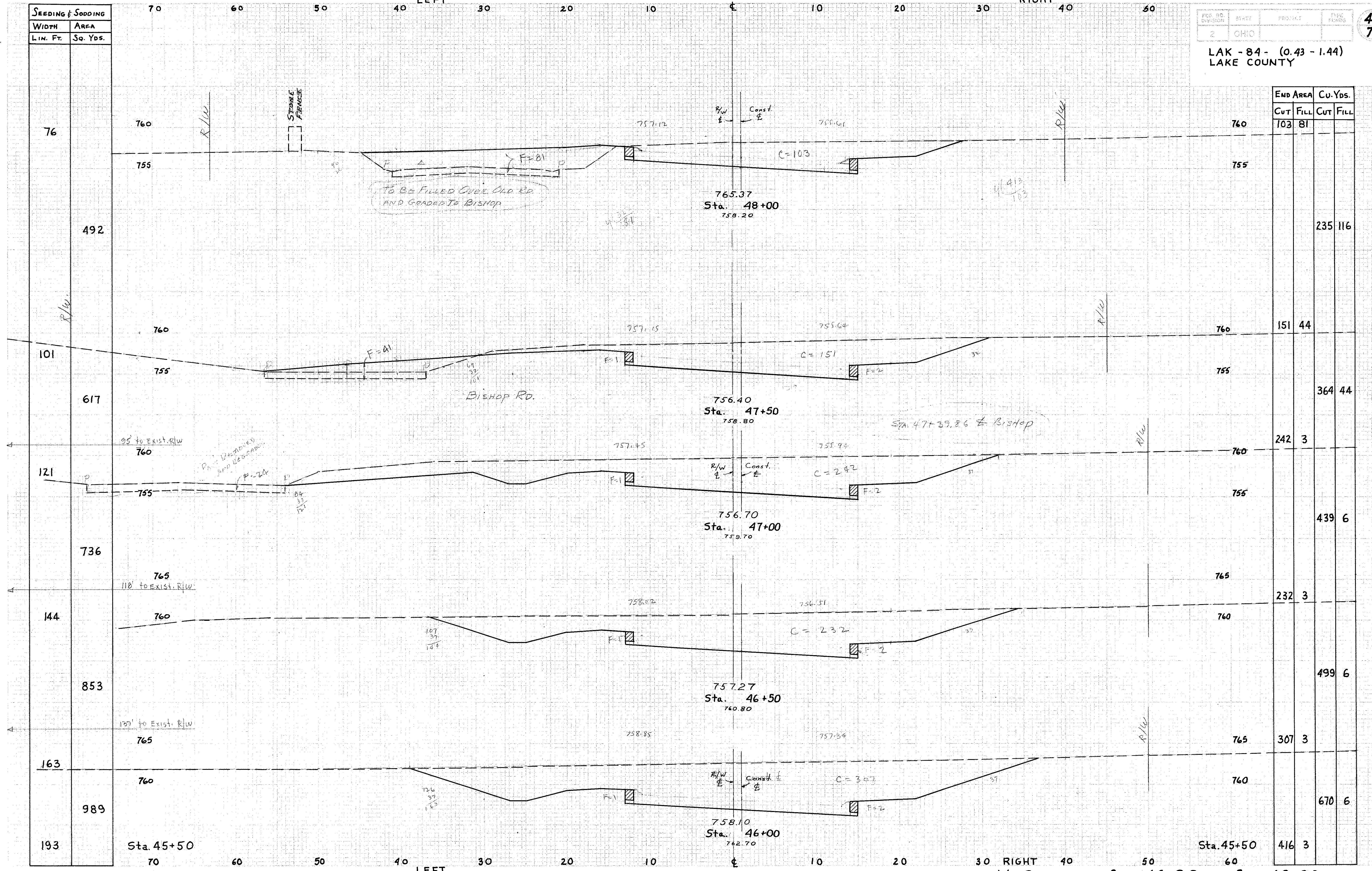
X-SECTIONS STA. 46+00 TO STA. 48+00
