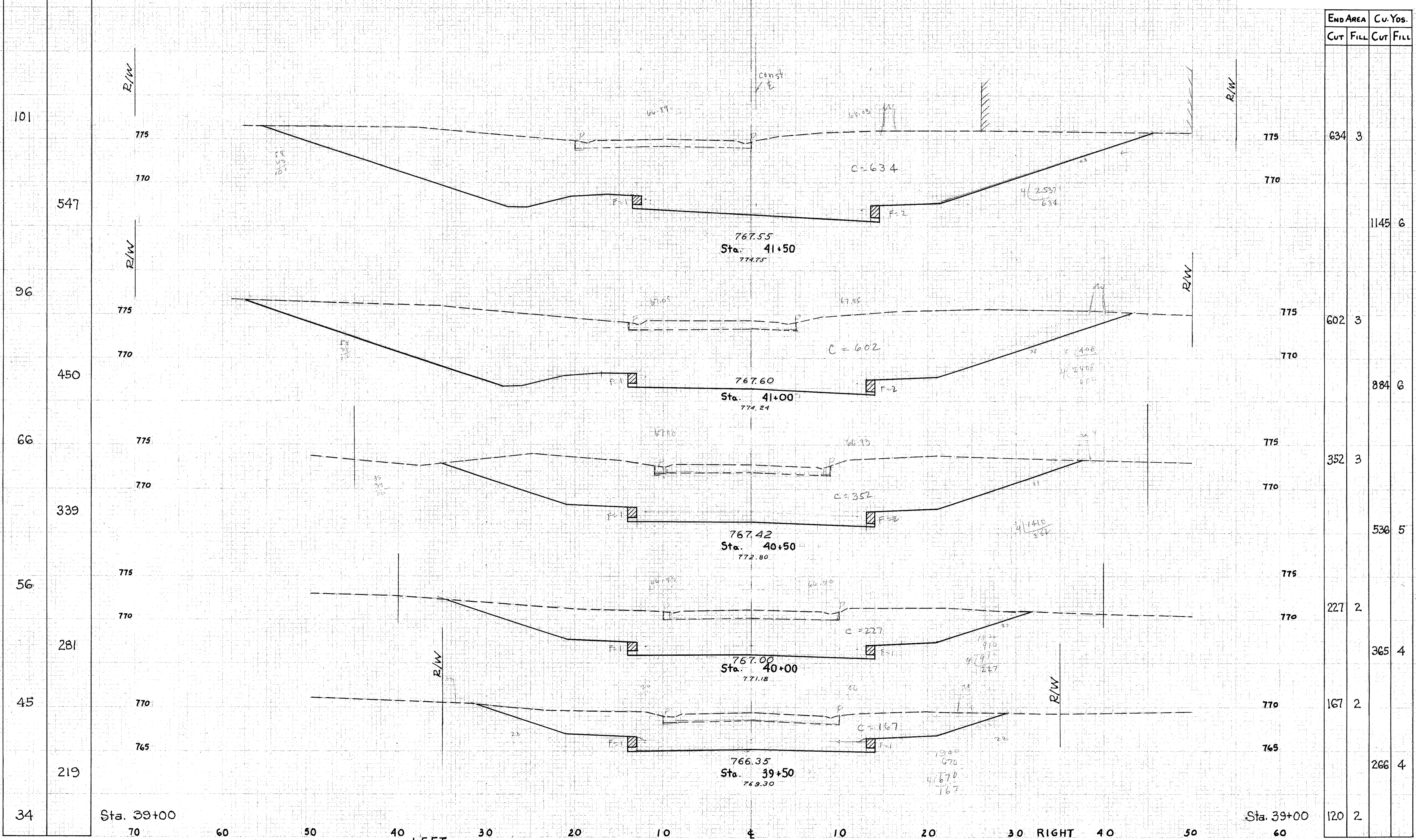
X-SECTIONS STA. 39+50 TO STA. 41+50
