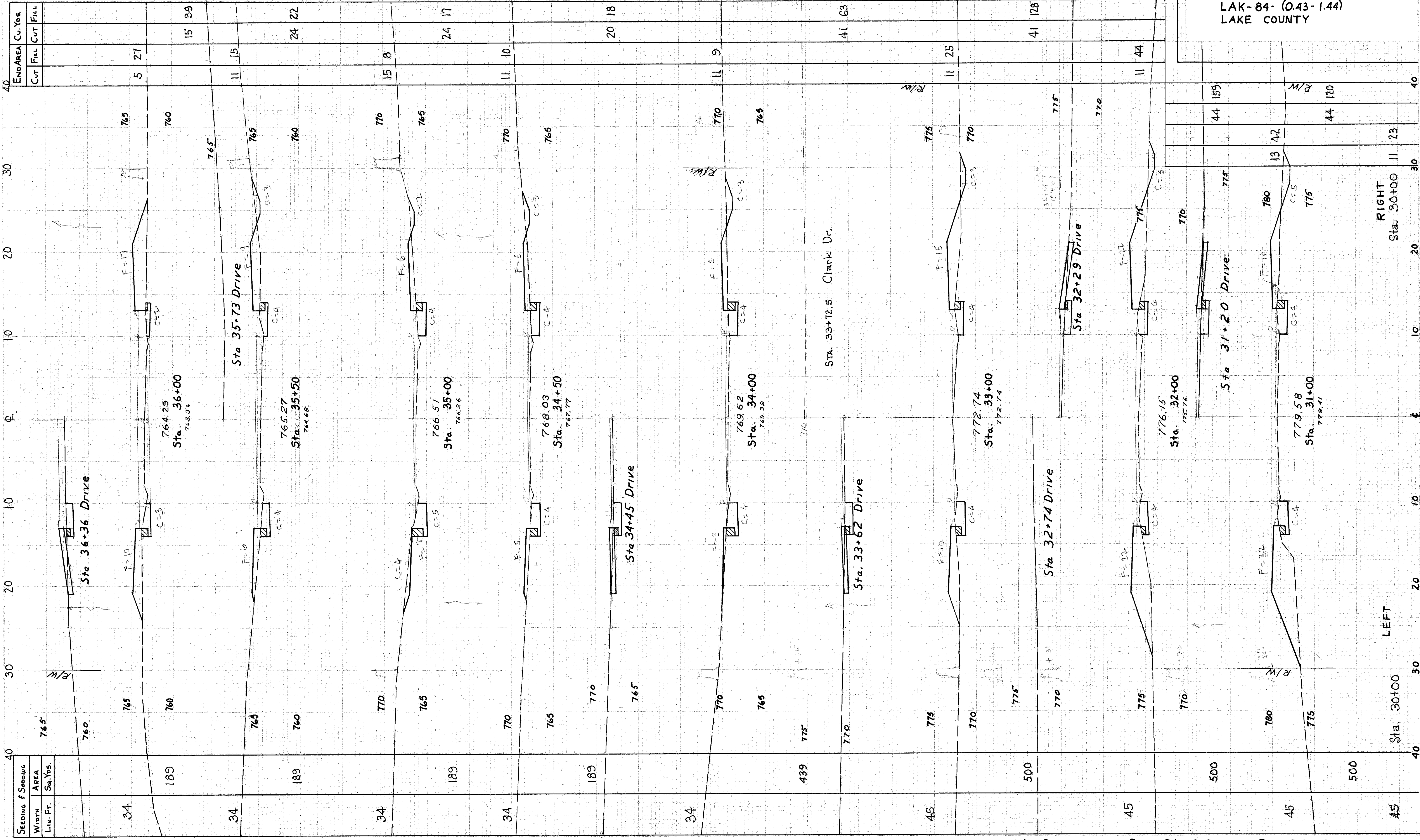
X-SECTIONS STA. 31+00 TO STA. 36+27
