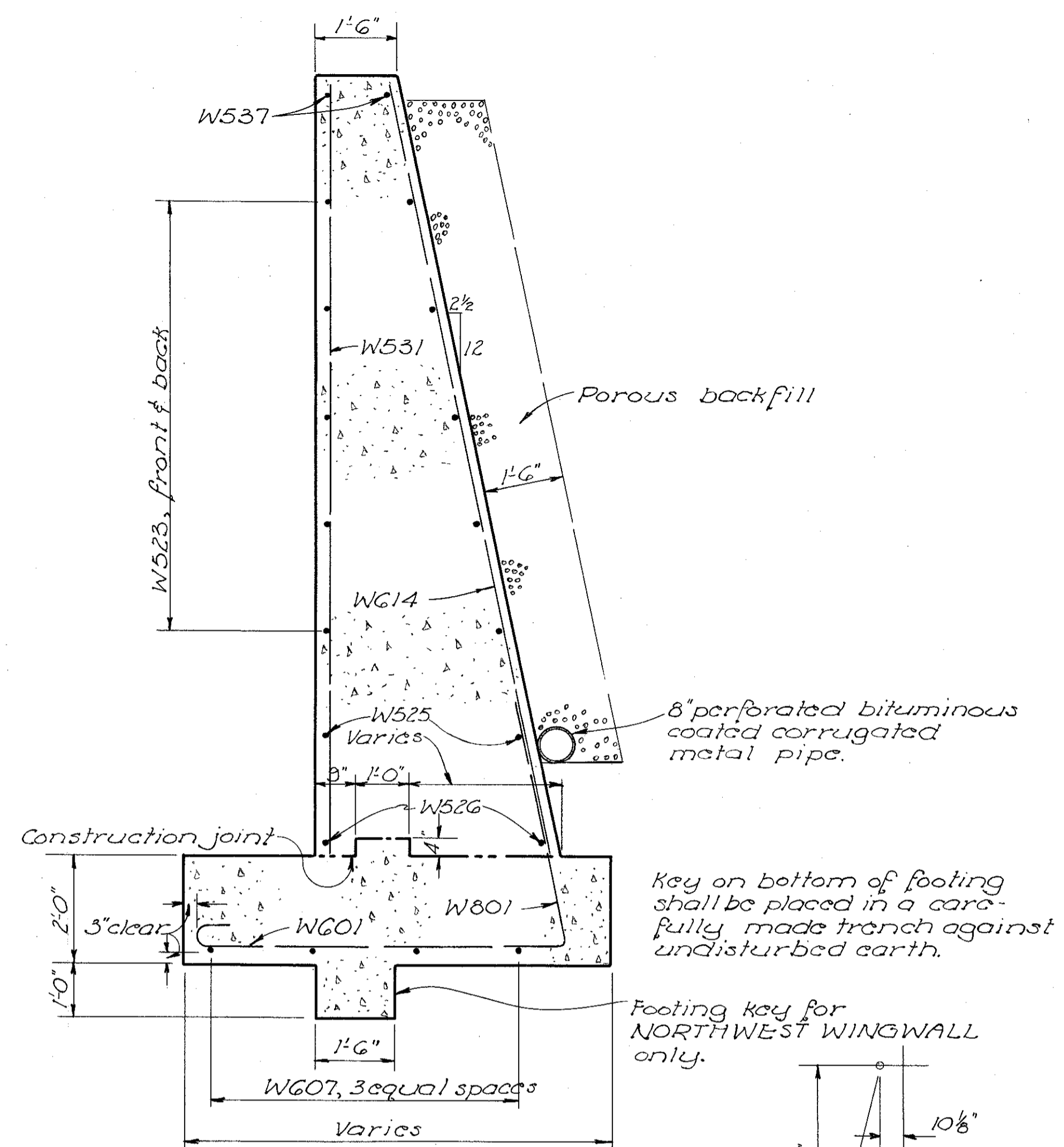
SECTION A-A
