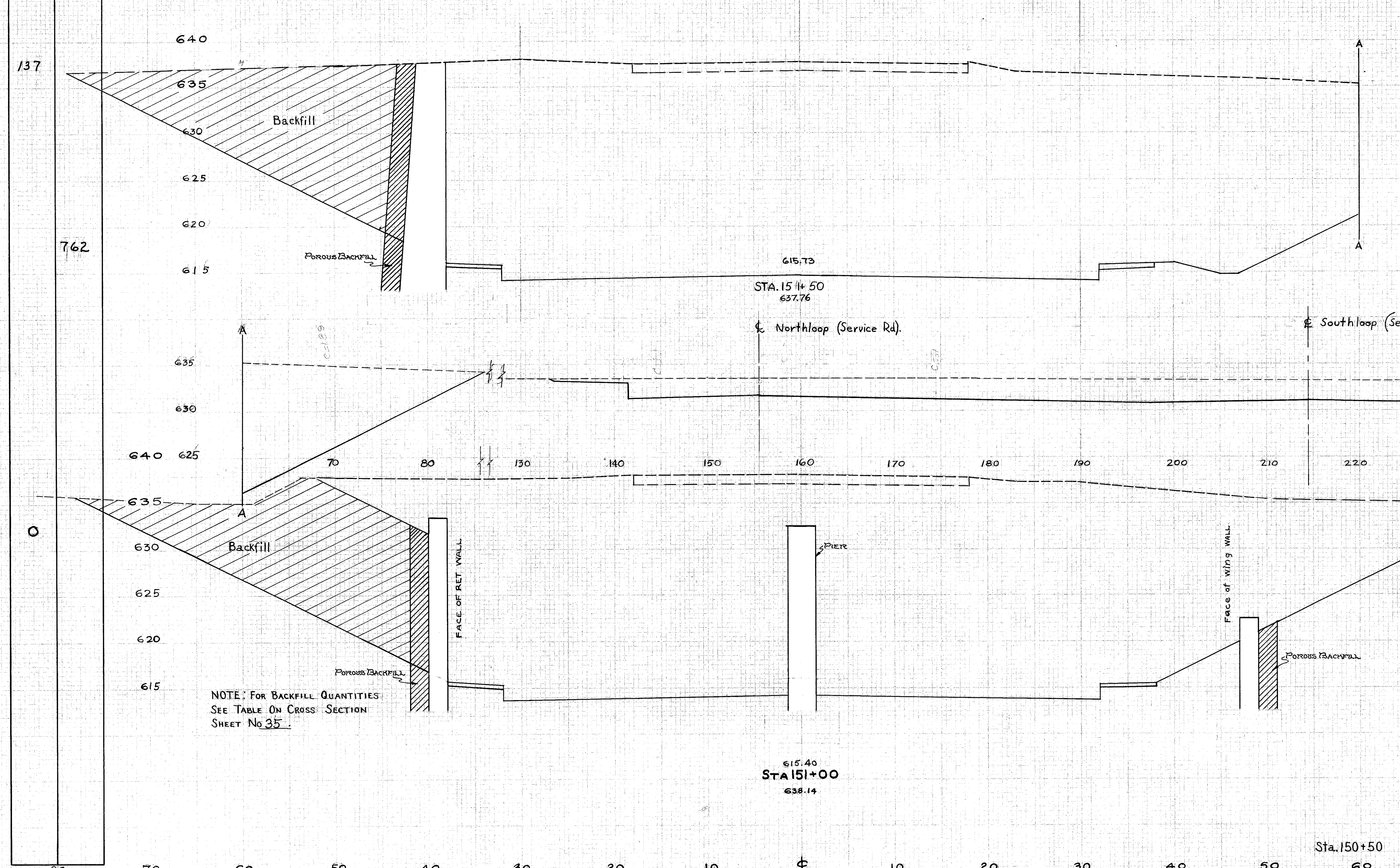
X-SECTIONS STA. 151+00 TO STA. 151+50
