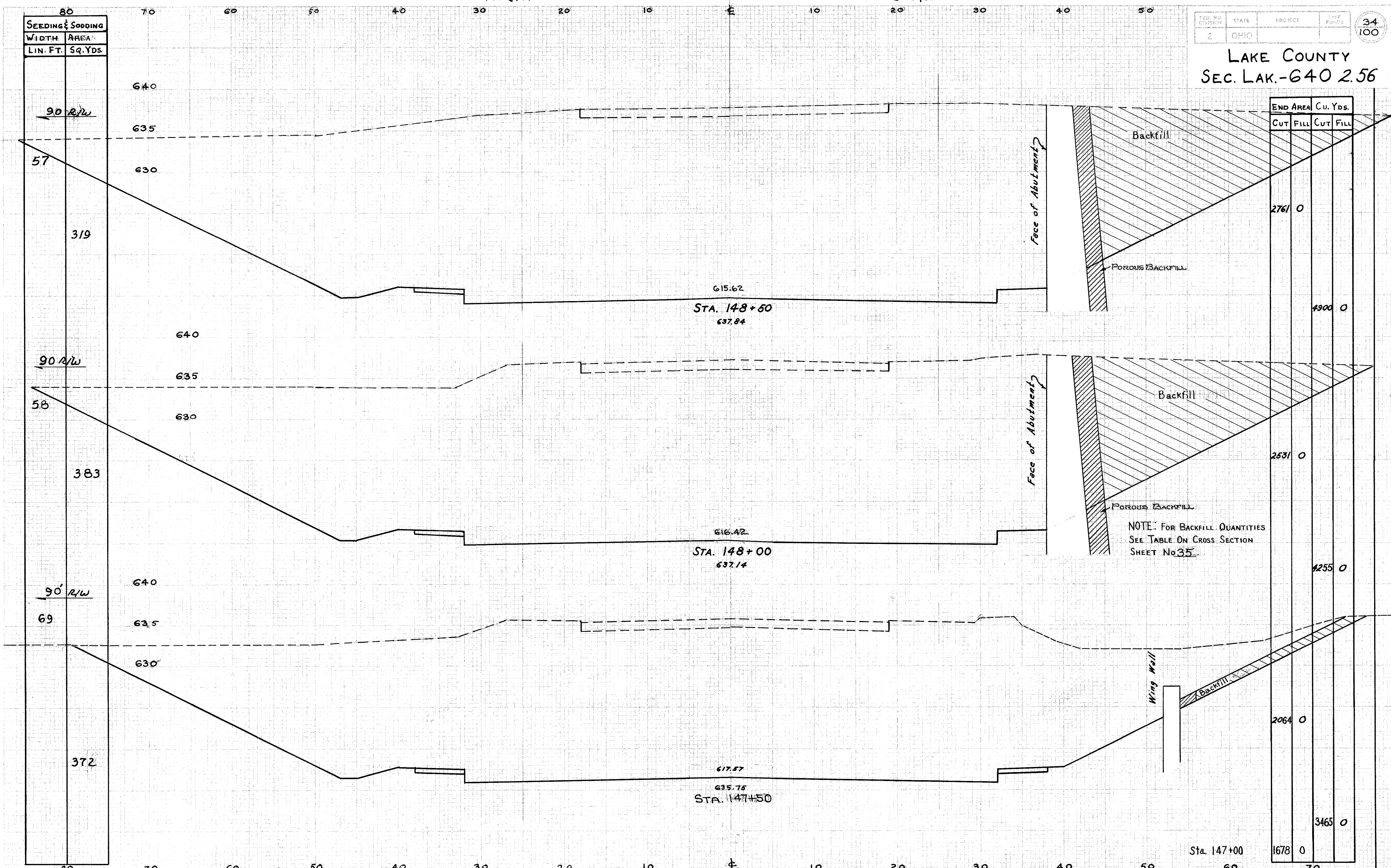
X-SECTIONS STA. 147+50 TO STA. 148+50
