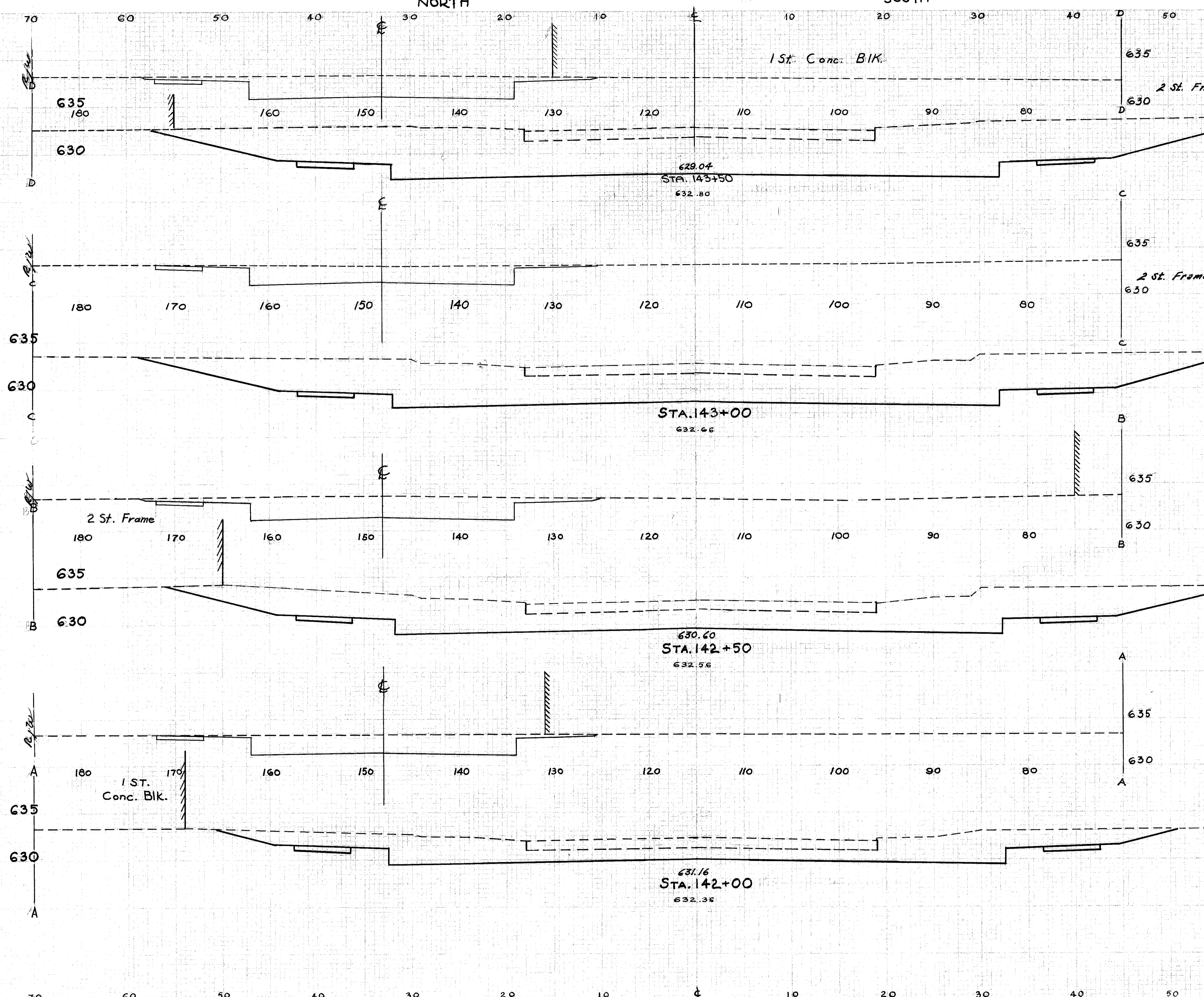
X-SECTIONS STA. 142+00 TO STA. 143+50
