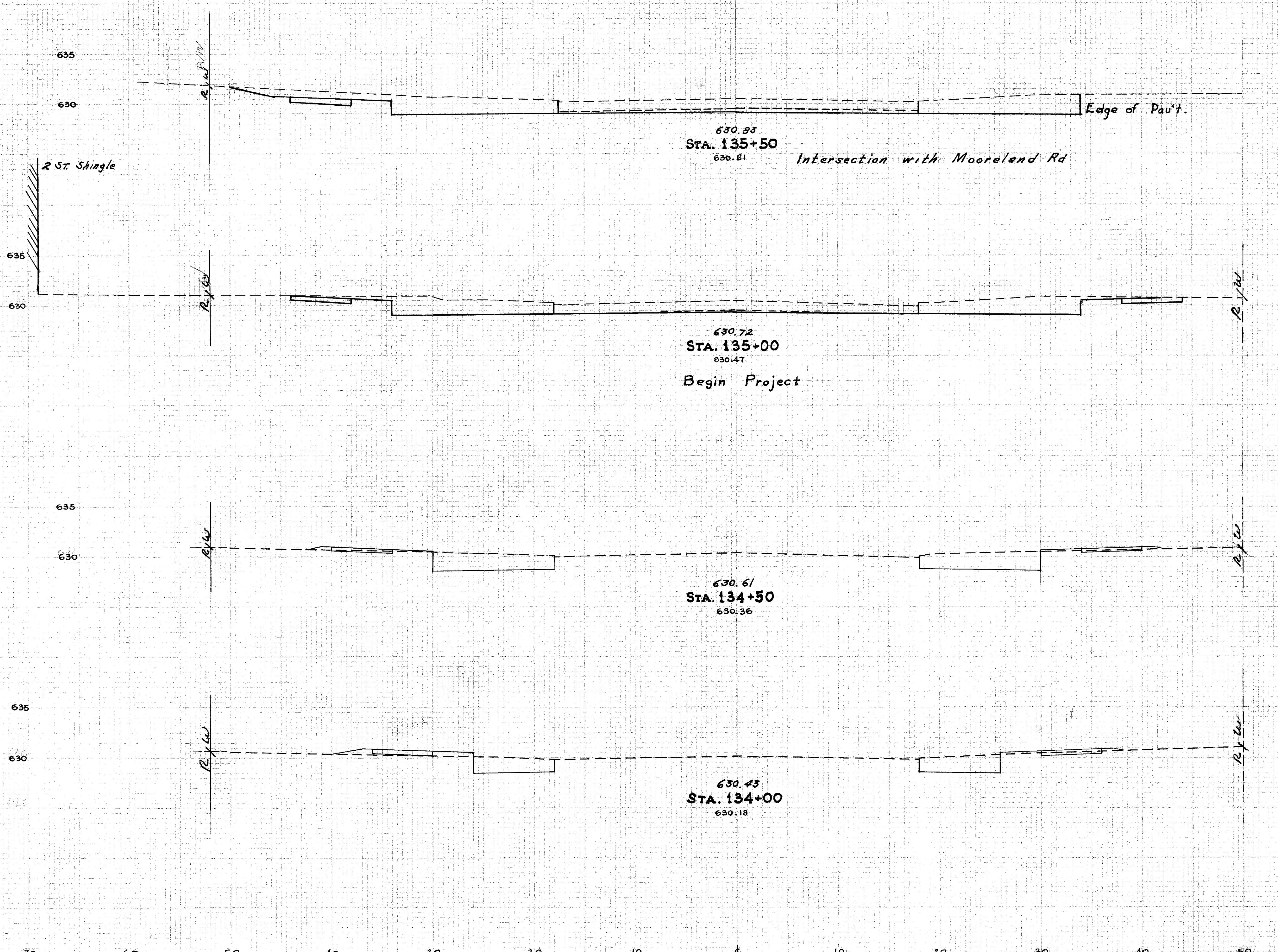
X-SECTIONS STA. 134+00 TO STA. 135+50
