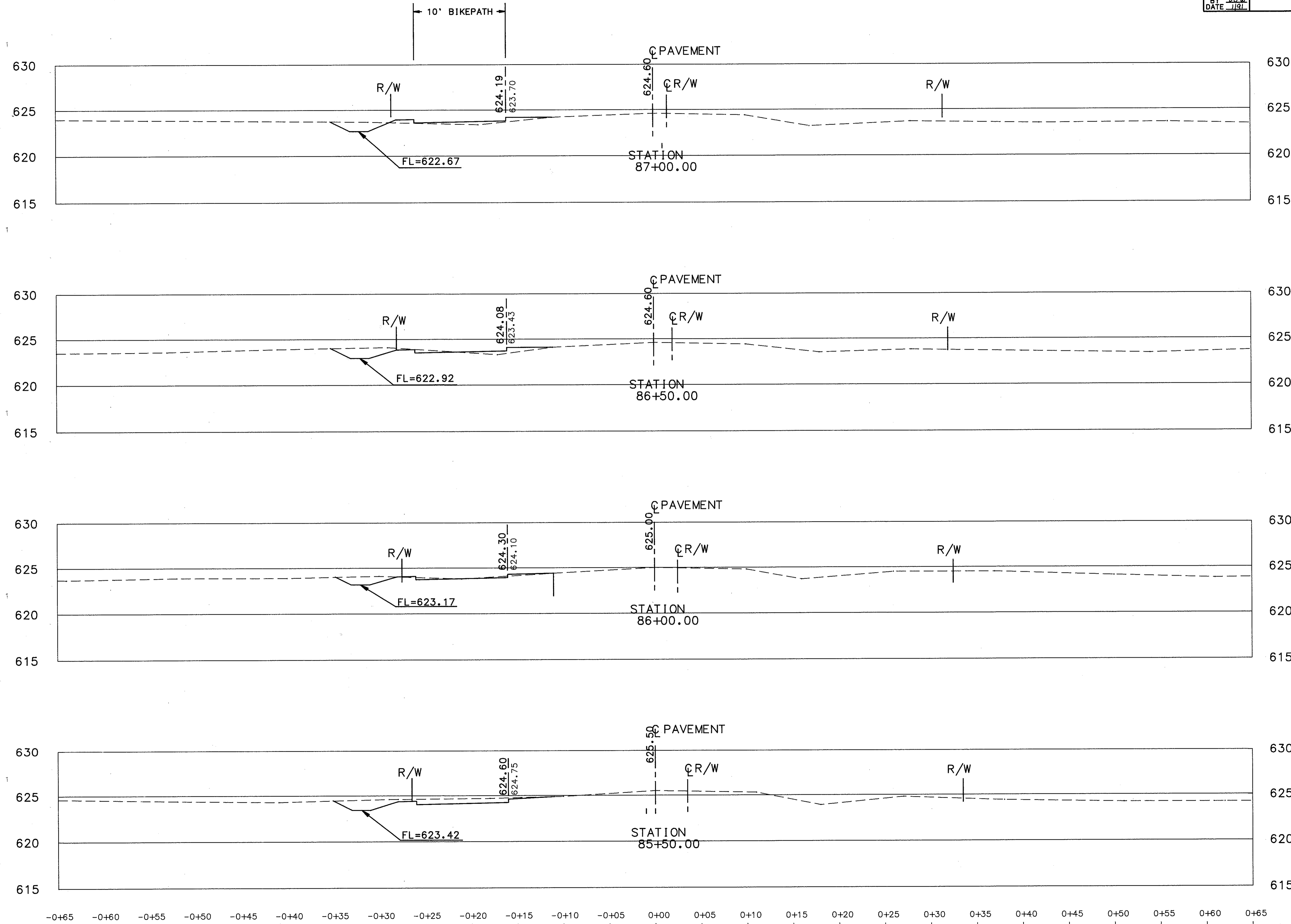
CROSS-SECTIONS STA. 85+50 TO STA. 87+00
