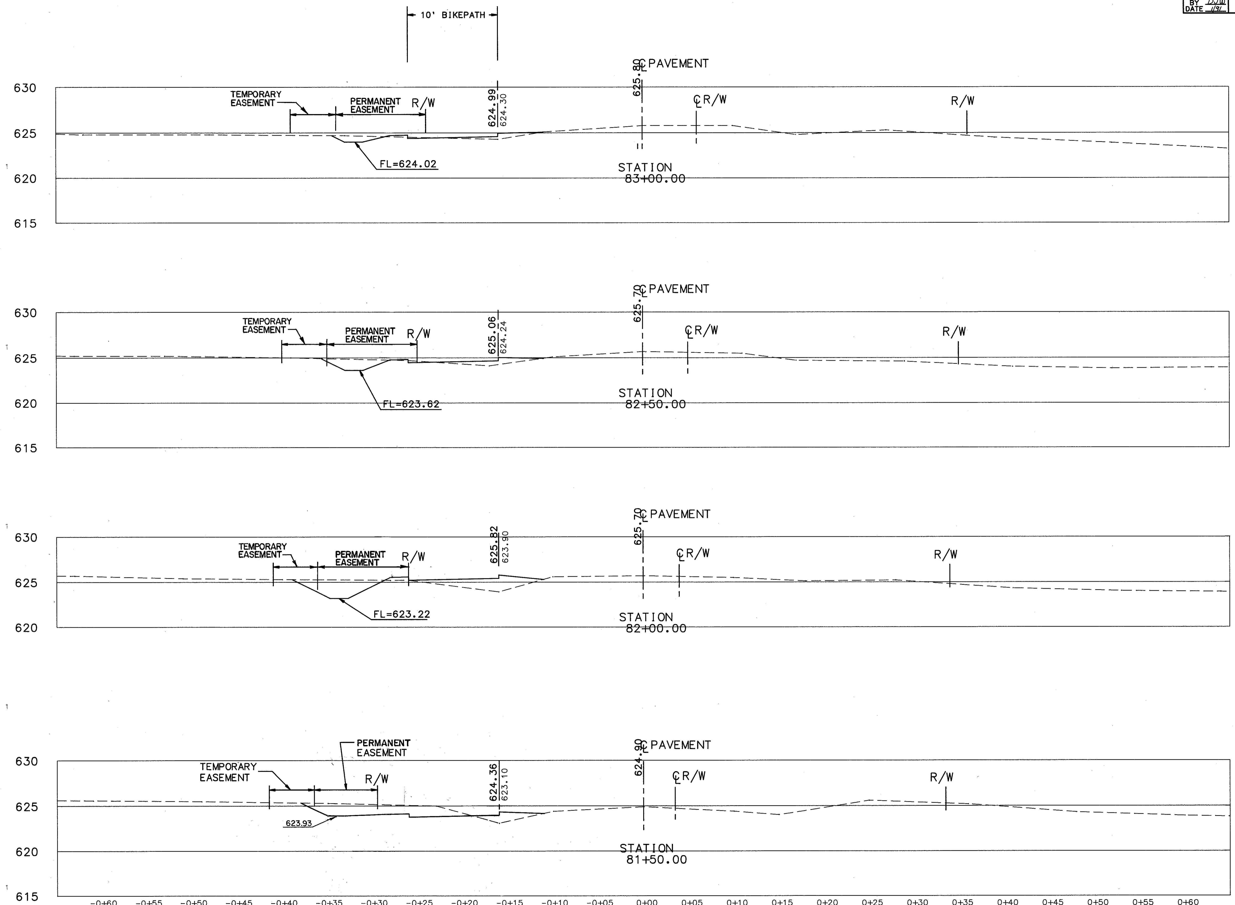
CROSS-SECTIONS STA. 81+50 TO STA. 83+00
