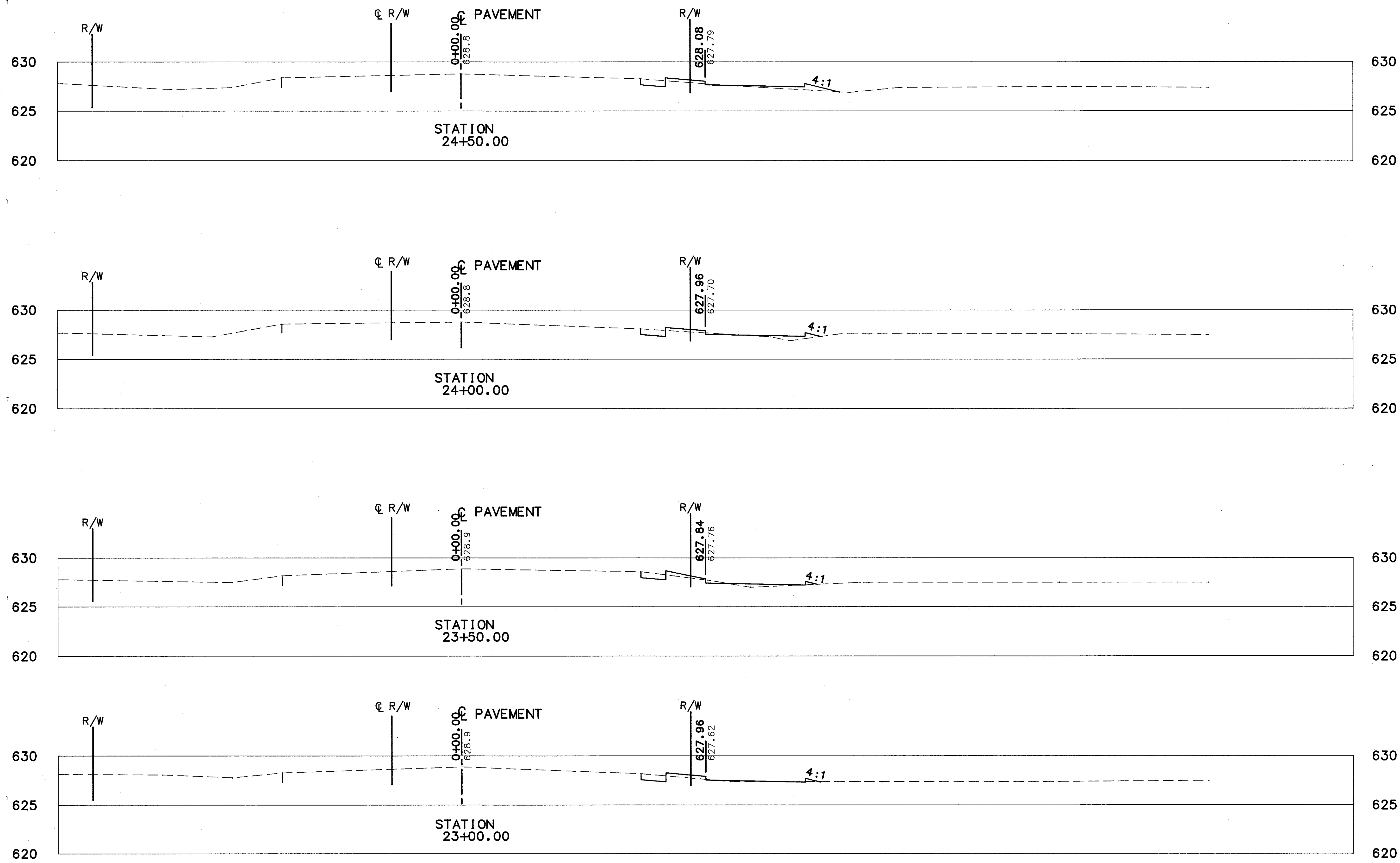
CROSS-SECTIONS STA. 23+00 TO STA. 24+50
