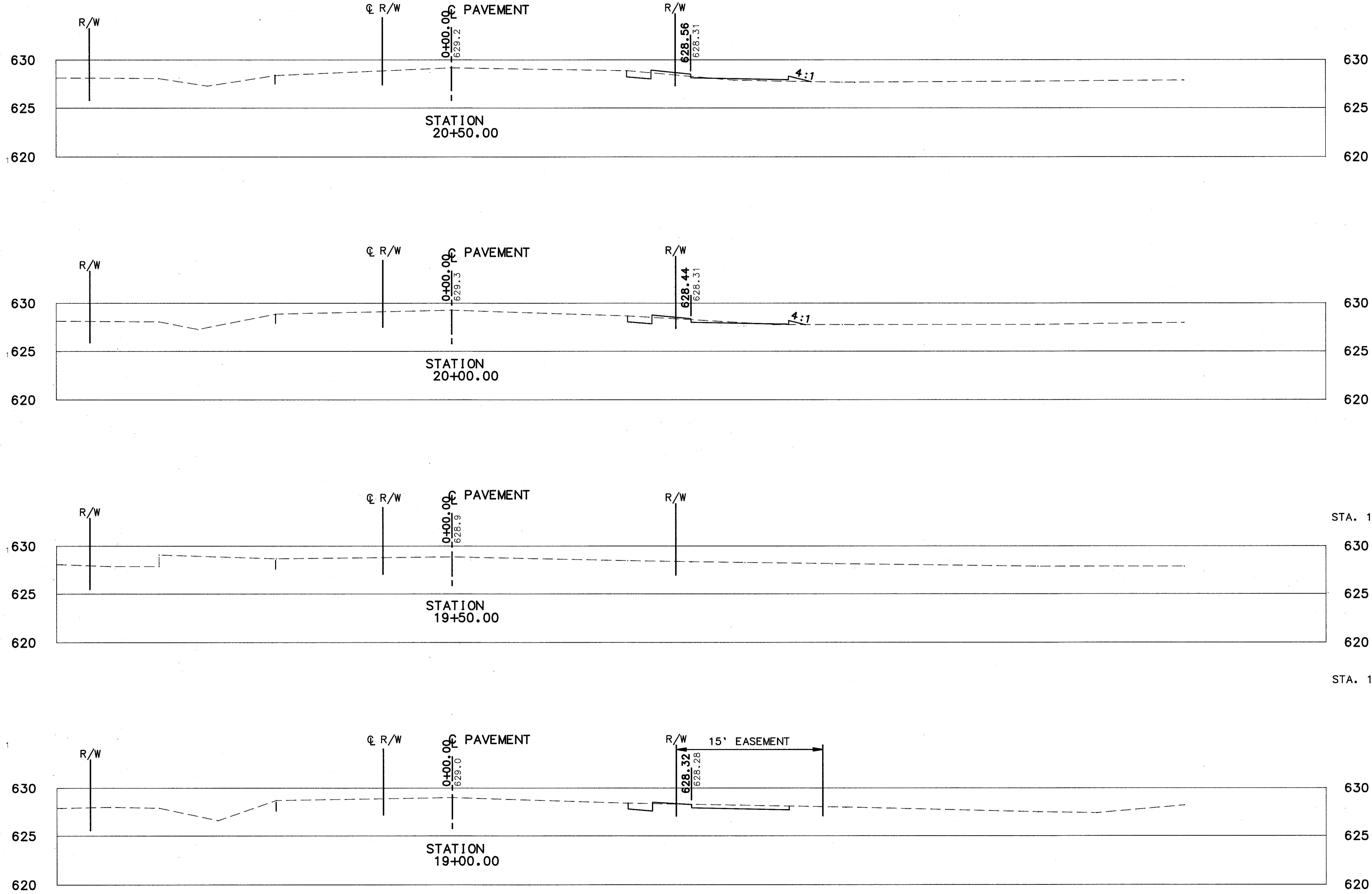
CROSS-SECTIONS STA. 19+00 TO STA. 20+50
