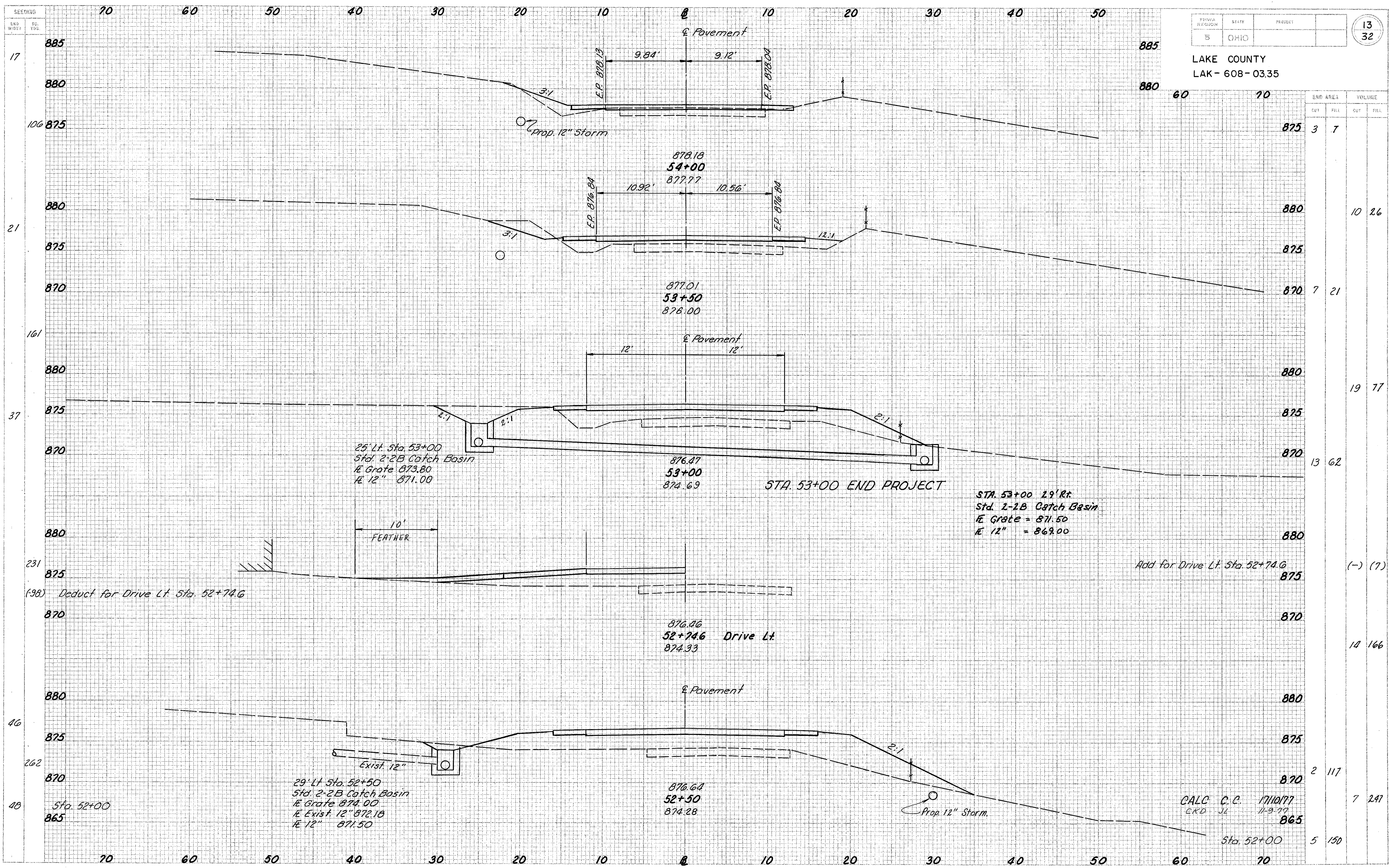
X-SECTIONS STA. 52+50 TO STA. 54+00
