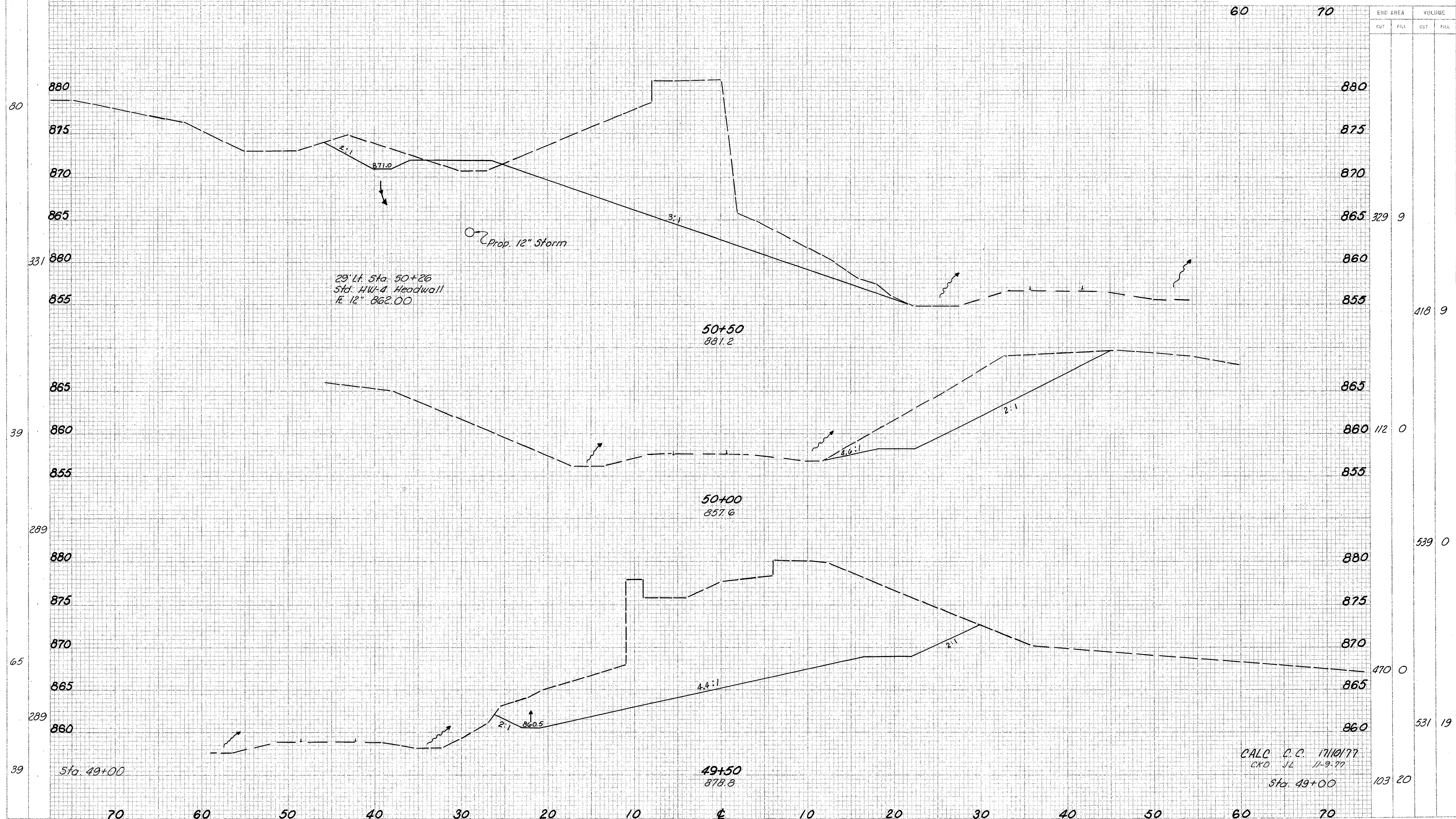
X-SECTIONS, STA. 49+50 to STA. 50+50
